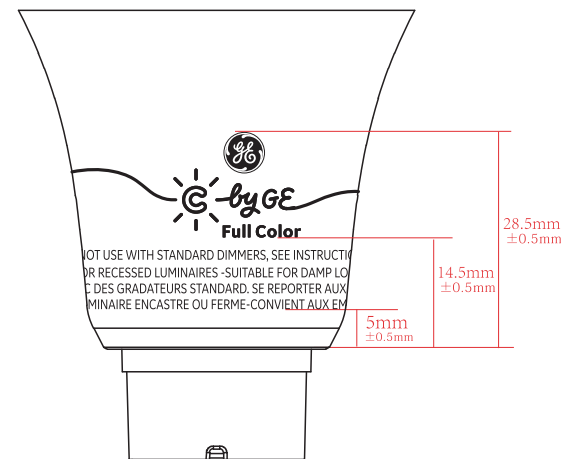
背面示意图
