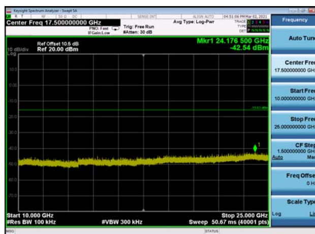
,Plot 5,10000MHz~25000MHz-802.11g ,2462MHz
