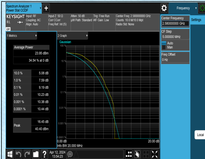
Band38-20MHz-QPSK-37850-1RB#0-PASS
