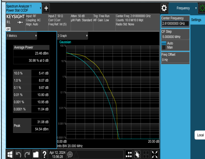
Band38-20MHz-QPSK-38150-1RB#0-PASS
