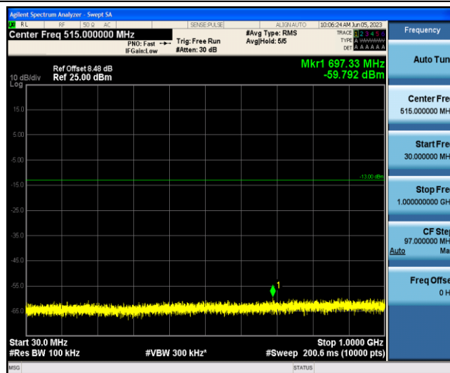
Band4-10MHz-QPSK-20350-1-0-Low-30-1000--59.79-PASS
