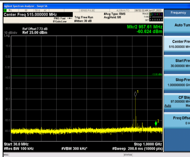
Band5-3MHz-QPSK-20415-1-0-Low-30-1000--60.62-PASS
