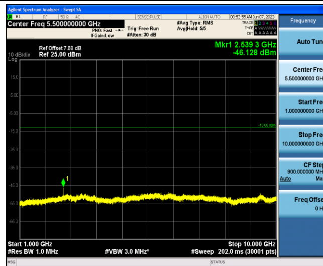
Band5-3MHz-QPSK-20635-1-0-Low-1000-10000--46.13-PASS
