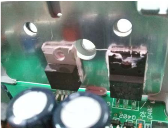
PC68LTD Main Audio IC
