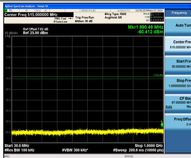
Band25-20MHz-16QAM-26365-1-0-Low-30-1000--60.41-PASS
