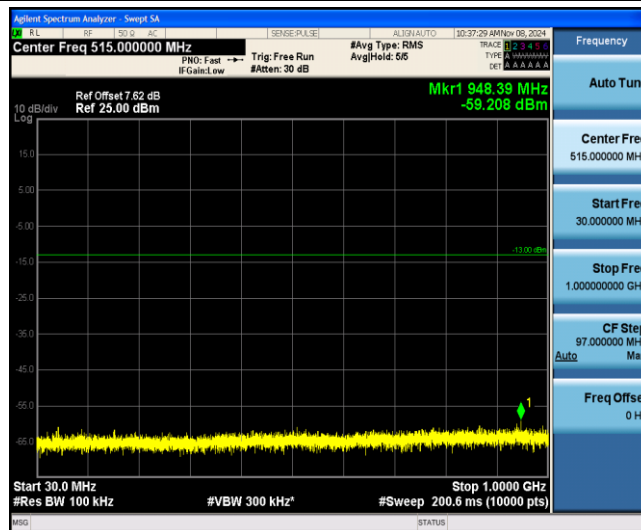
Band25-10MHz-16QAM-26090-1-0-Low-30-1000--59.21-PASS
