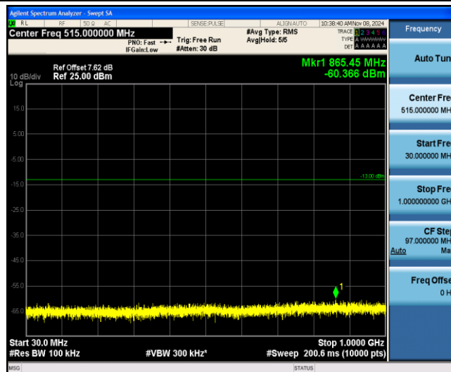
Band25-10MHz-16QAM-26365-1-0-Low-30-1000--60.37-PASS
