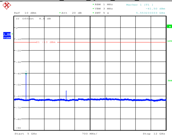
Band2_20MHz_QPSK_18700_1RB#0
