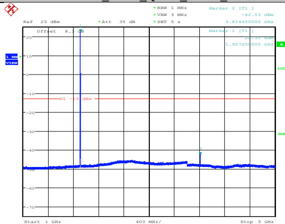
Band2_3MHz_QPSK_19185_1RB#0
