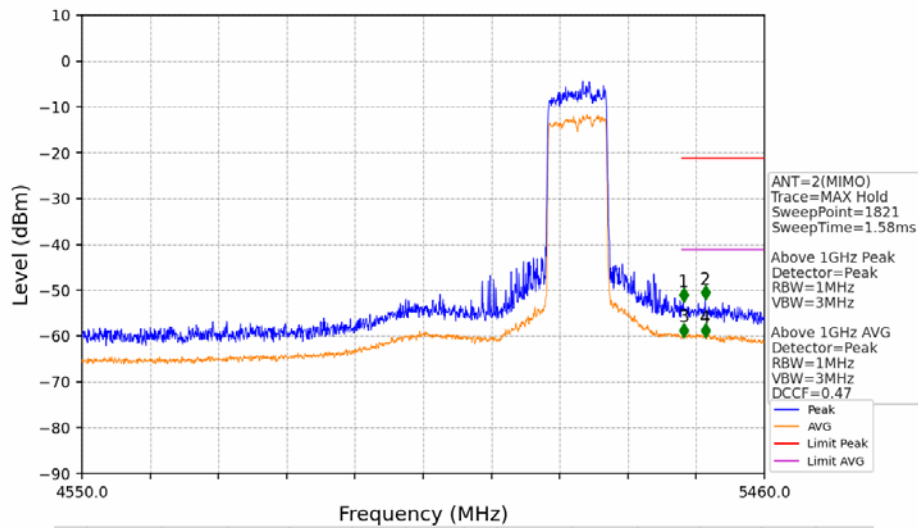
802.11ax(HEW80)_MCH_5210MHz_RU996_Left_Ant2_NTNV
