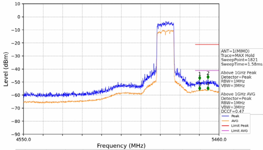
802.11ax(HEW80)_MCH_5210MHz_RU996_Left_Ant1_NTNV
