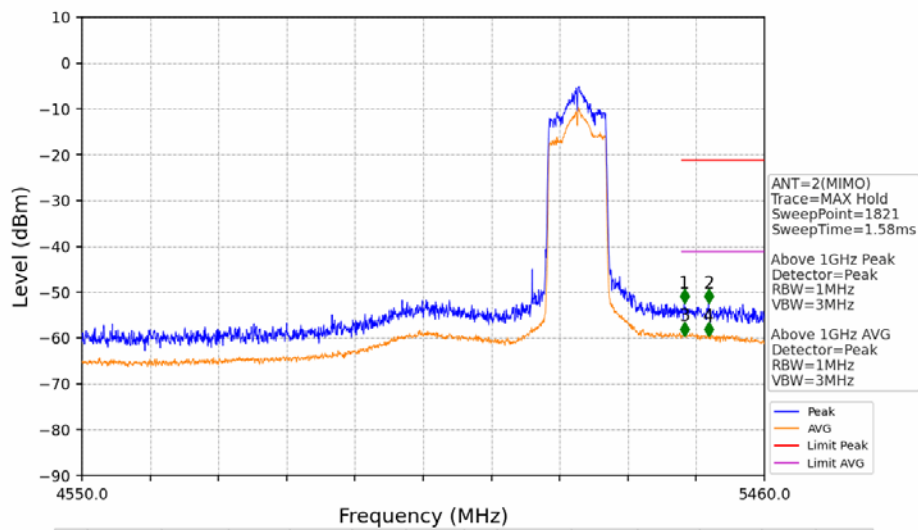
802.11ac(VHT80)_MCH_5210MHz_Ant2_NTNV
