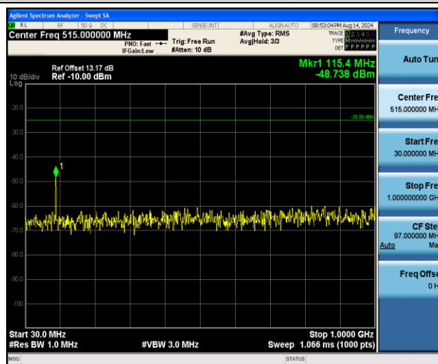
Band41-15MHz-QPSK-41515-1RB#0-Range4:1000~3000MHz
