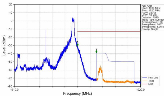
Band25 5MHz QPSK HCH 1912.5MHz RB 1 24 NTV
