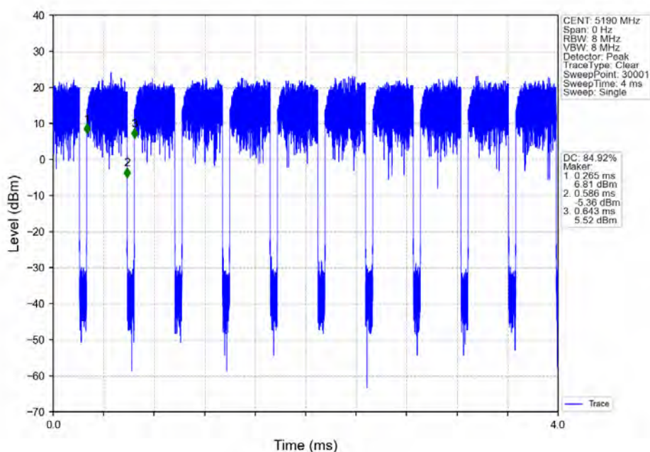
802.11ax(HE40)_LCH_5190MHz_RU484_Left_Ant2_NTNV
