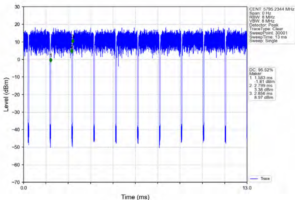
802.11ax(HE80) MCH_5775MHz_RU484_Right_Ant2_NTNV
