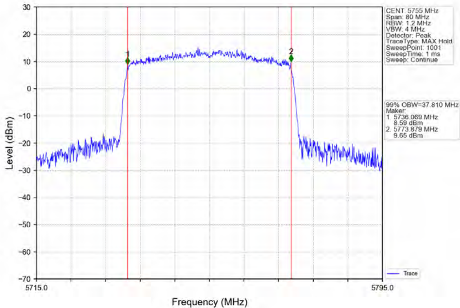
802.11ax(HE40)_LCH_5755MHz_RU484_Left_Ant2_NTNV
