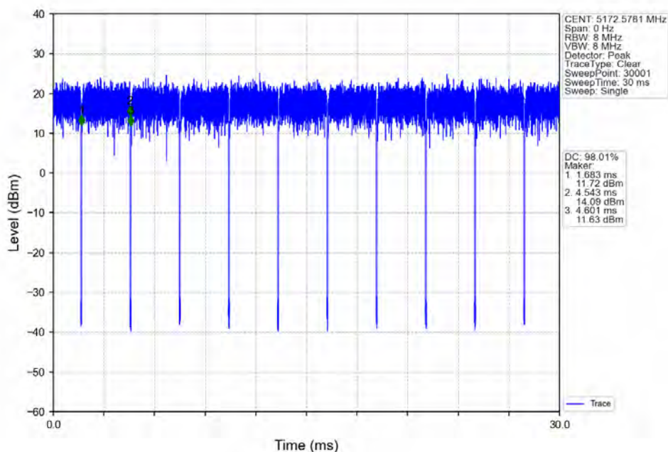
802.11ax(HE20)_LCH_5180MHz_RU52_Left_Ant2_NTNV
