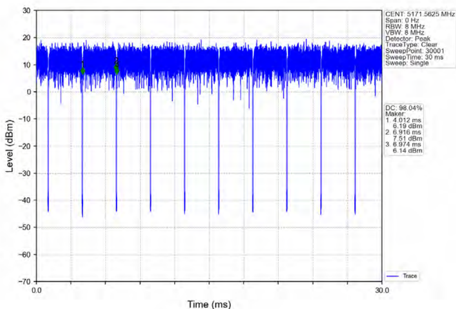
802.11ax(HE20)_LCH_5180MHz_RU26_Left_Ant2_NTNV
