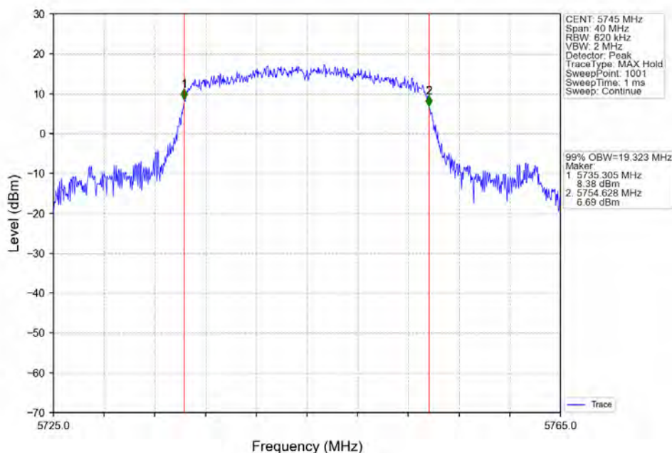
802.11ax(HE20)_LCH_5745MHz_RU242_Left_Ant2_NTNV
