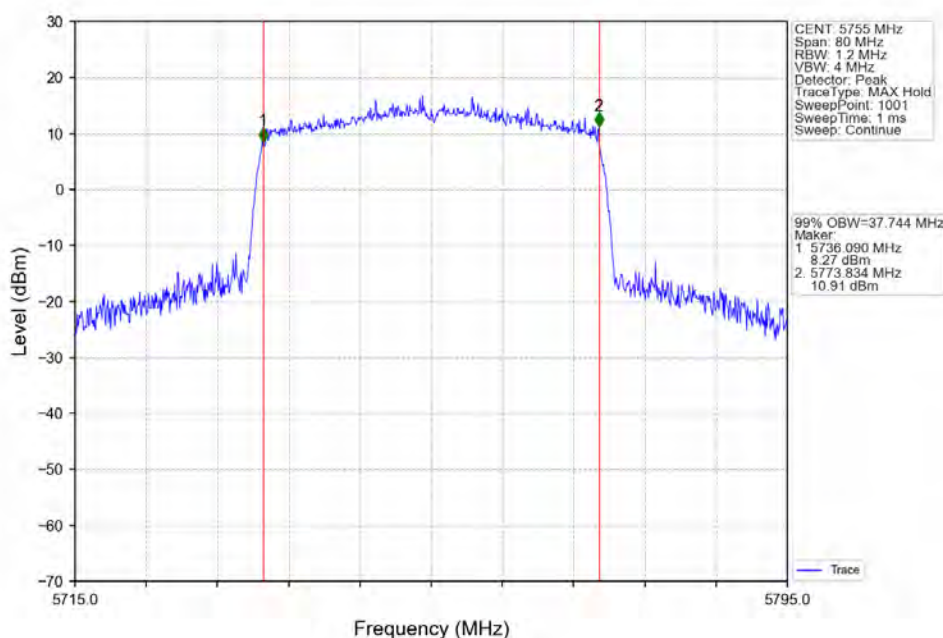
802.11ax(HE40)_LCH_5755MHz_RU484_Left_Ant1_NTNV
