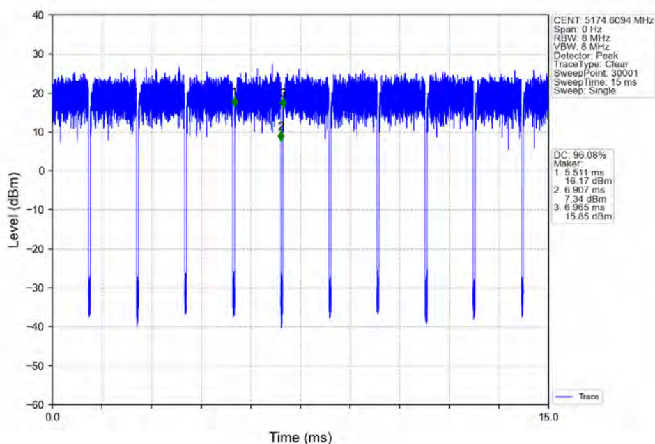
802.11ax(HE20)_LCH_5180MHz_RU106_Left_Ant1_NTNV
