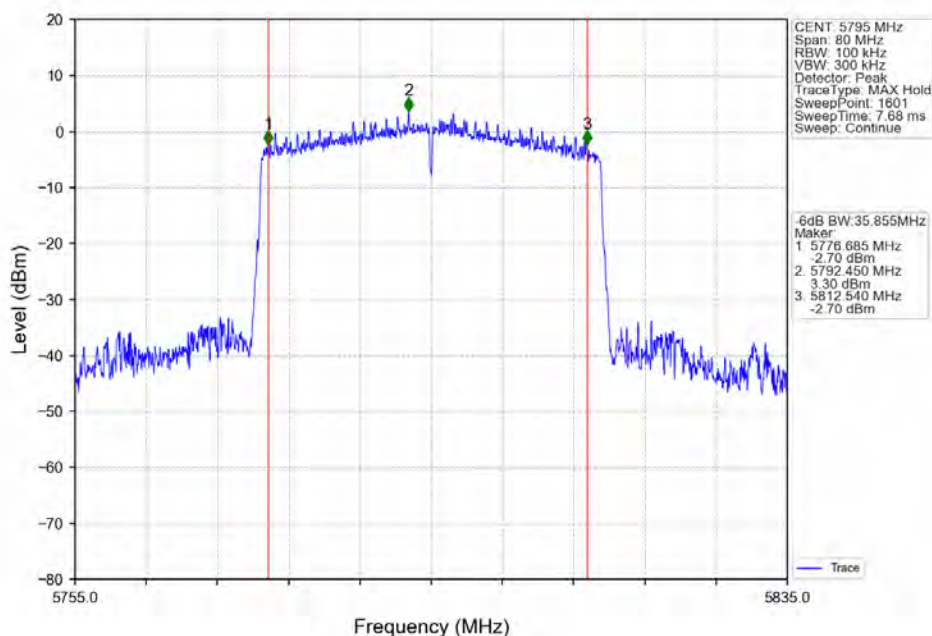
802.11ax(HE40)_HCH_5795MHz_RU484_Left_Ant2_NTNV
