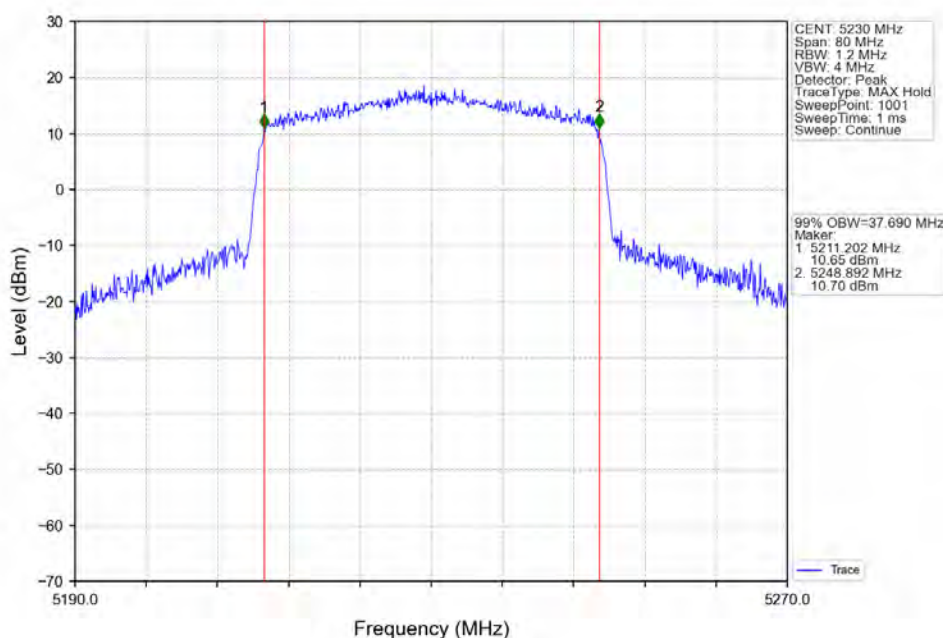
802.11ax(HE40)_HCH_5230MHz_RU484_Left_Ant2_NTNV
