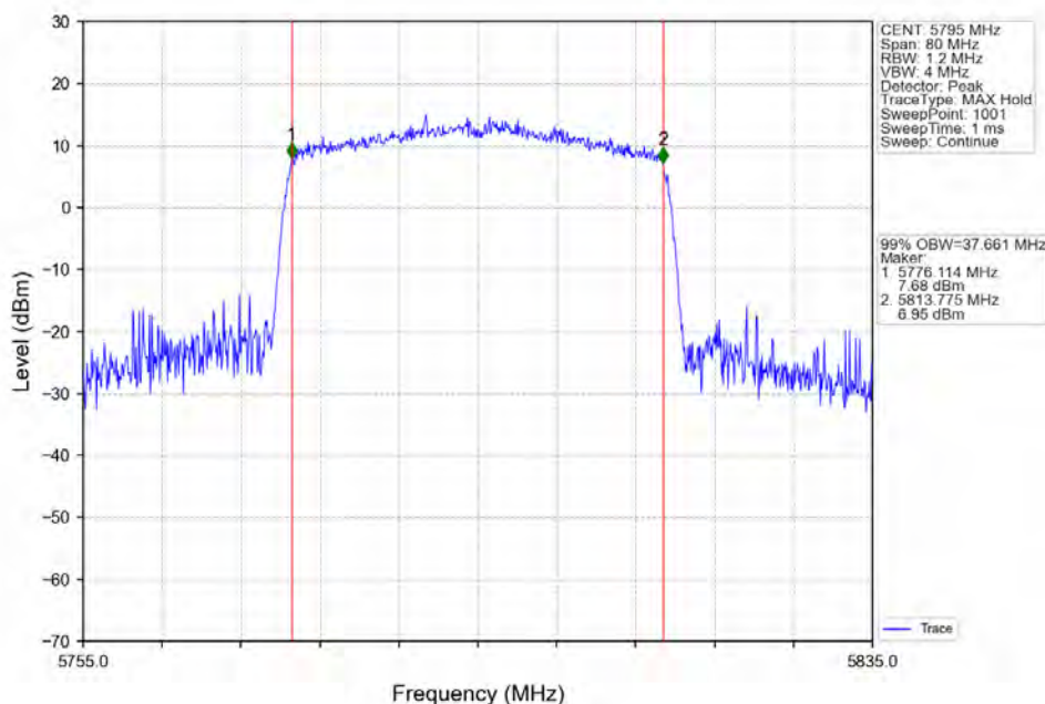
802.11ax(HE40)_HCH_5795MHz_RU484_Left_Ant2_NTNV
