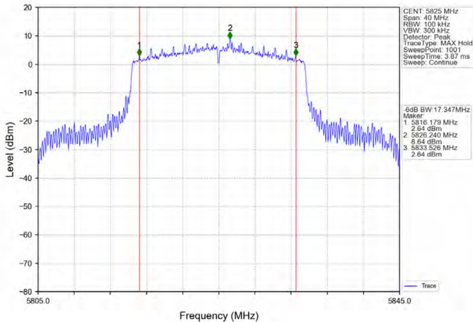
802.11ax(HE20)_HCH_5825MHz_RU242_Left_Ant2_NTNV
