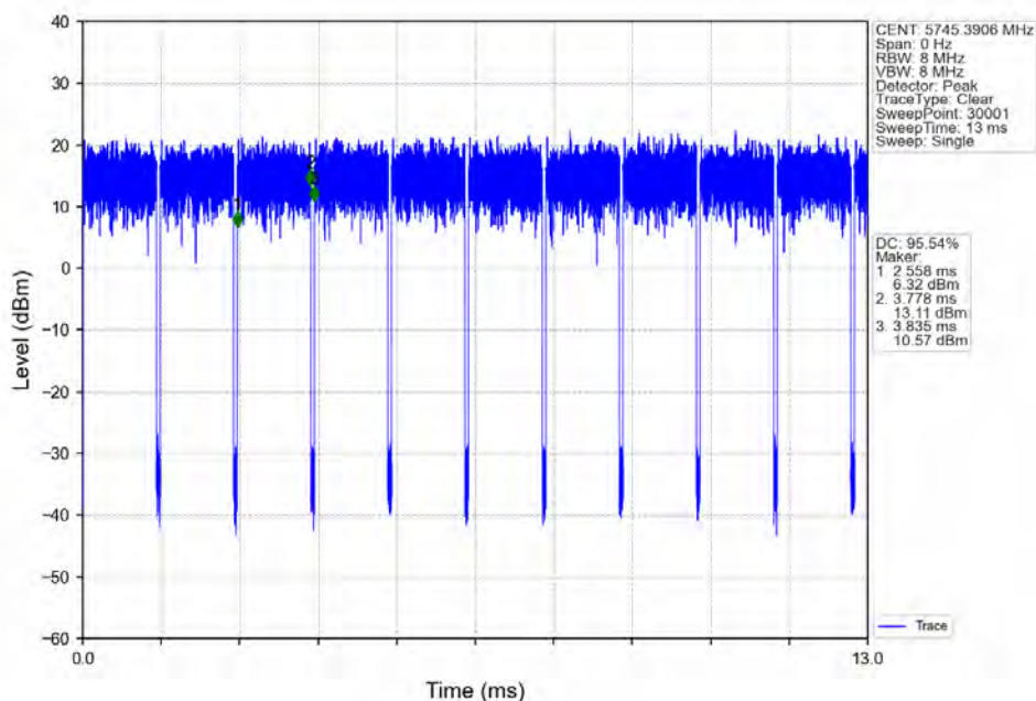
802.11ax(HE40)_LCH_5755MHz_RU242_Left_Ant2_NTNV
