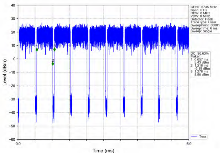
802.11ax(HE20)_LCH_5745MHz_RU242_Left_Ant2_NTNV
