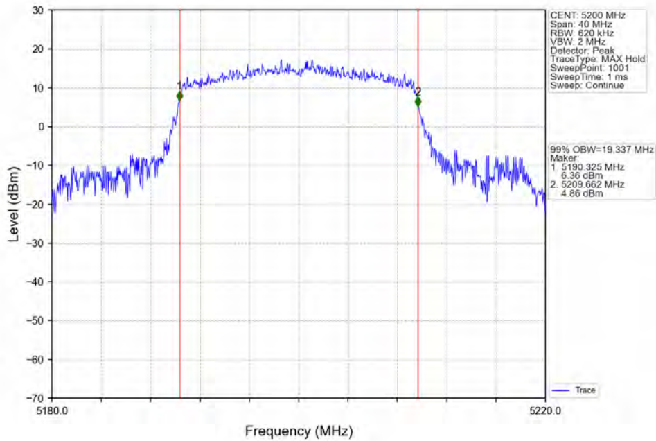
802.11ax(HE20)_MCH_5200MHz_RU242_Left_Ant1_NTNV
