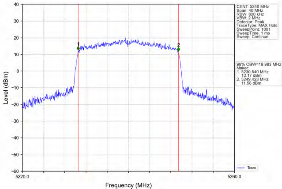
802.11ax(HE20)_HCH_5240MHz_RU242_Left_Ant2_NTNV
