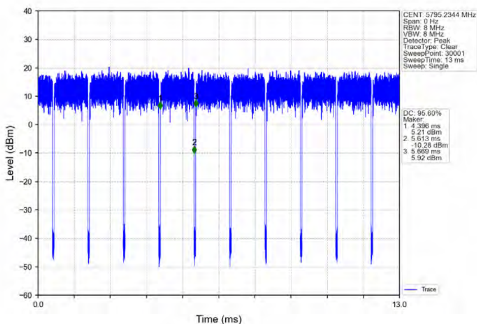
802.11ax(HE80)_MCH_5775MHz_RU484_Right_Ant1_NTNV
