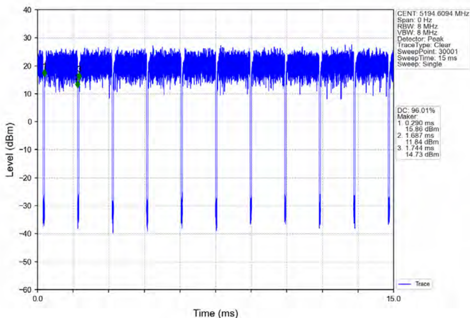
802.11ax(HE20)_MCH_5200MHz_RU106_Left_Ant2_NTNV
