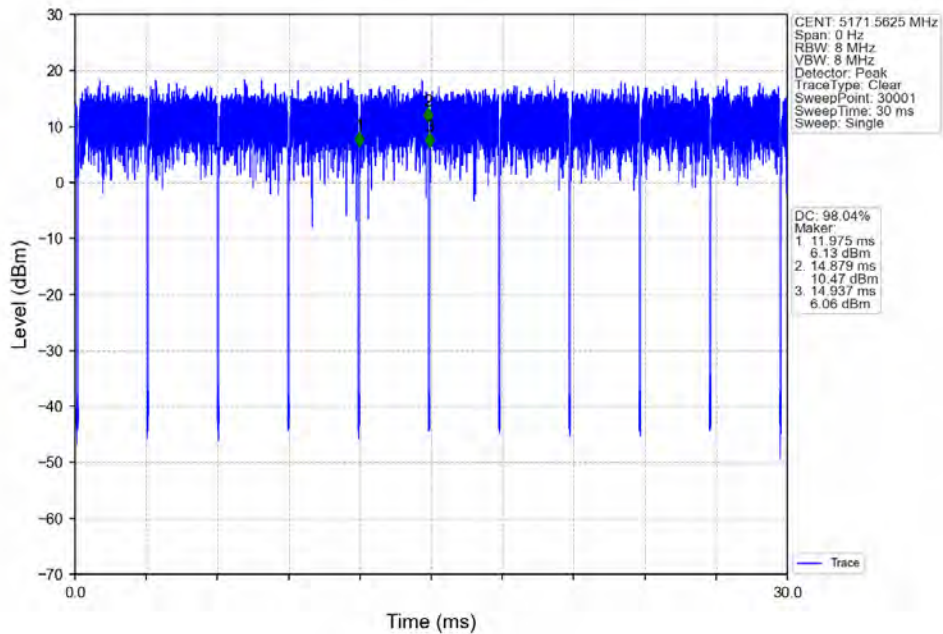
802.11ax(HE20)_LCH_5180MHz_RU26_Left_Ant1_NTNV
