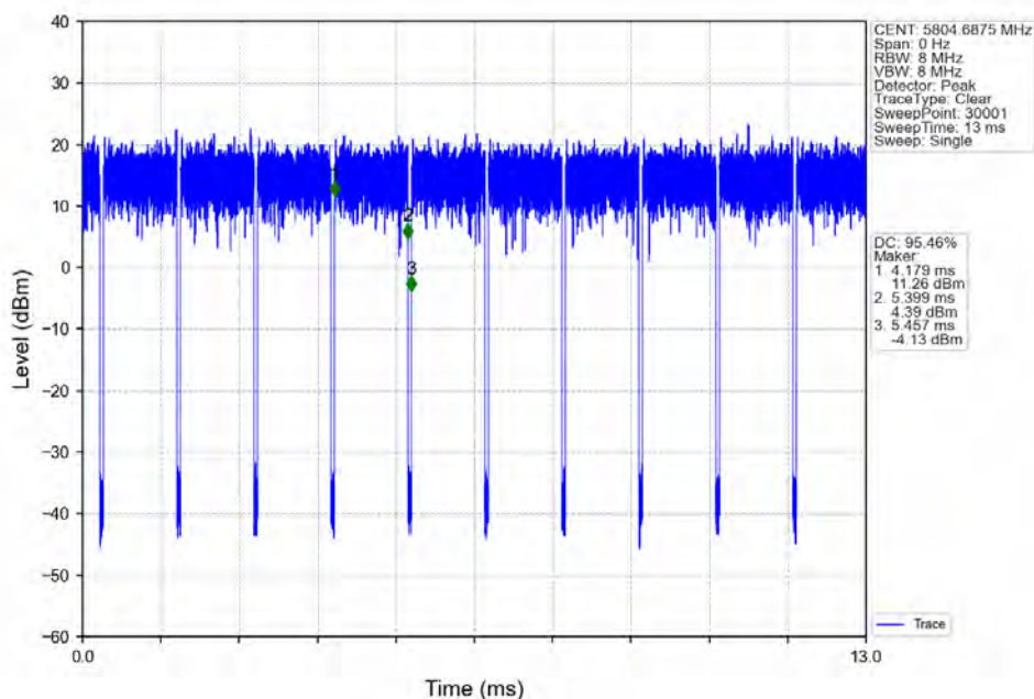
802.11ax(HE40)_HCH_5795MHz_RU242_Right_Ant2_NTNV
