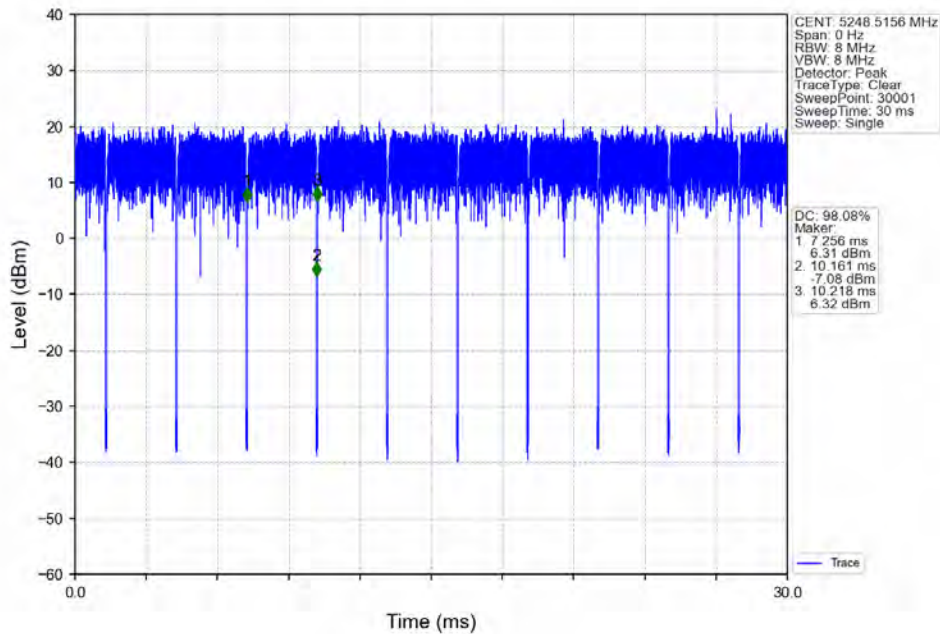
802.11ax(HE20)_HCH_5240MHz_RU26_Right_Ant1_NTNV
