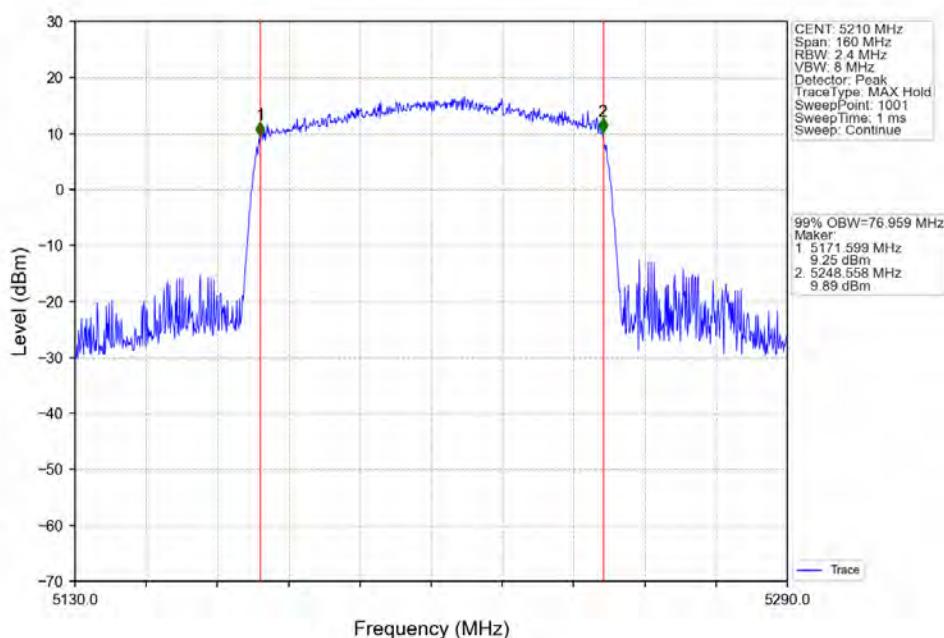
802.11ax(HE80)_MCH_5210MHz_RU996_Left_Ant2_NTNV
