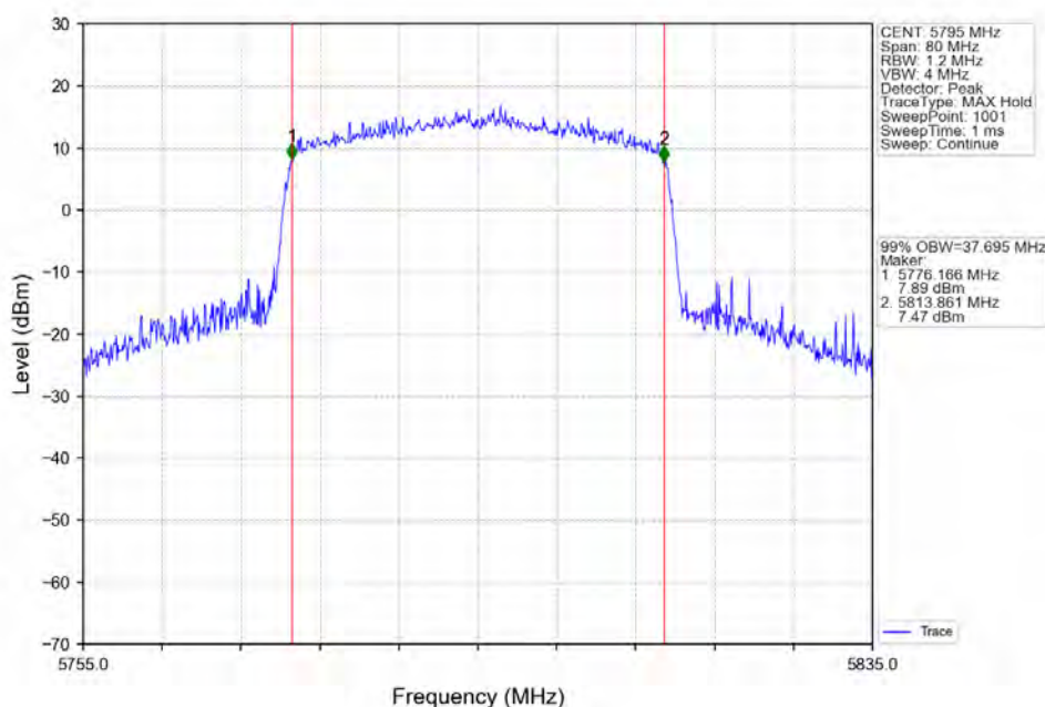
802.11ax(HE40)_HCH_5795MHz_RU484_Left_Ant1_NTNV
