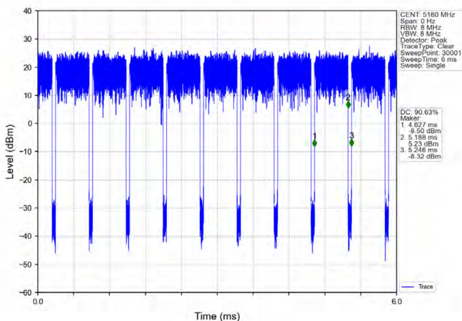
802.11ax(HE20)_LCH_5180MHz_RU242_Left_Ant2_NTNV
