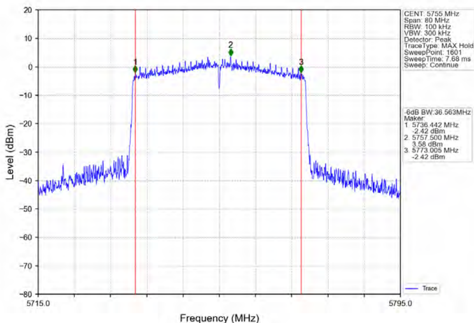
802.11ax(HE40)_LCH_5755MHz_RU484_Left_Ant2_NTNV
