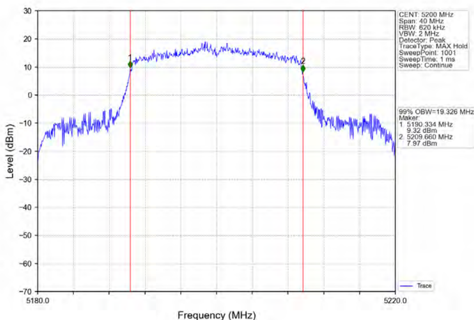
802.11ax(HE20)_MCH_5200MHz_RU242_Left_Ant2_NTNV
