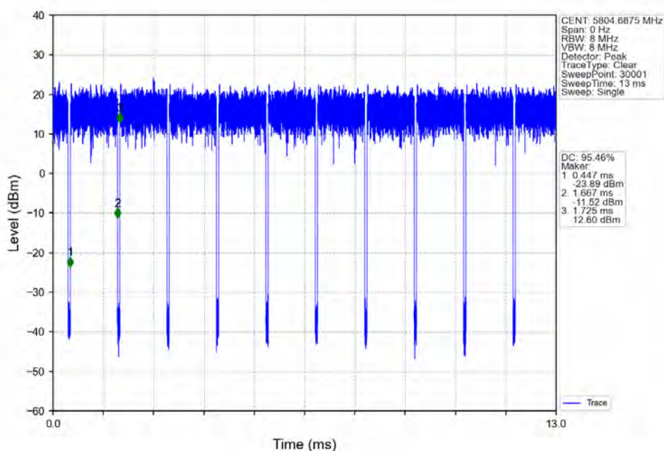
802.11ax(HE40) HCH_5795MHz_RU242_Right_Ant1_NTNV
