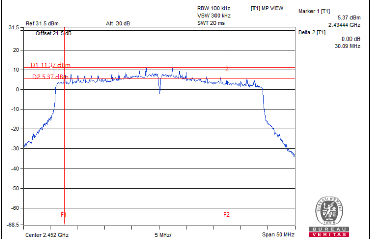
802.11be (EHT40) Beamforming / Chain 0 : CH 9
