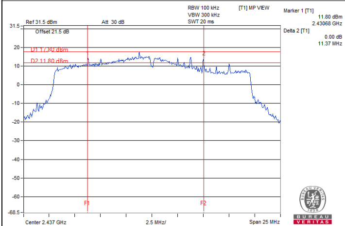
802.11be (EHT20) Beamforming / Chain 1 : CH 6
