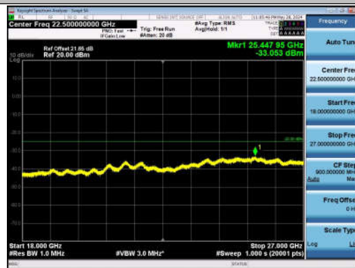
7-7-20MHz-20MHz-QPSK-QPSK-21152-21350-1RB#0-0RB #0-18000~27000MHz-PASS
