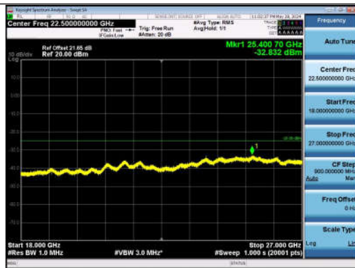
7-7-20MHz-20MHz-QPSK-QPSK-21001-21199-1RB#0-0RB #0-18000~27000MHz-PASS
