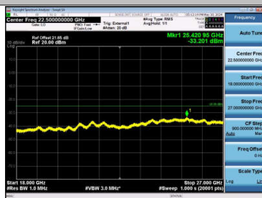
41-41-20MHz-20MHz-QPSK-QPSK-40340-40538-1RB#0-0 RB#0-18000~27000MHz-PASS
