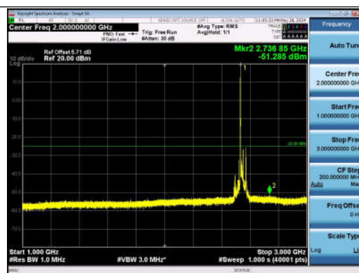
7-7-20MHz-20MHz-QPSK-QPSK-21152-21350-1RB#0-0RB #0-1000~3000MHz-PASS
