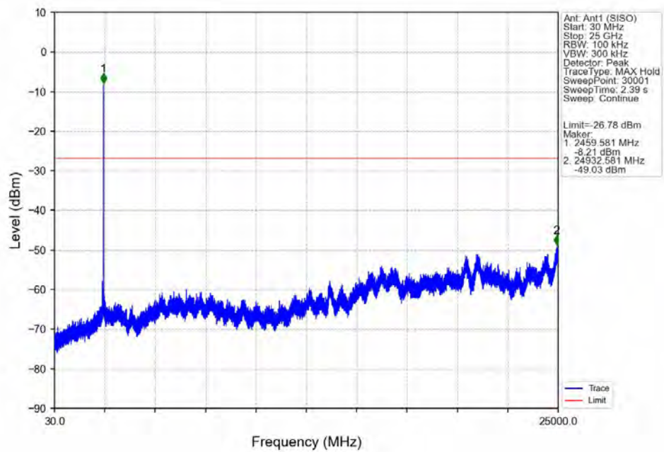
802.11ax(HEW20)_HCH_2462MHz_Ant1 (SISO)_NTNV
