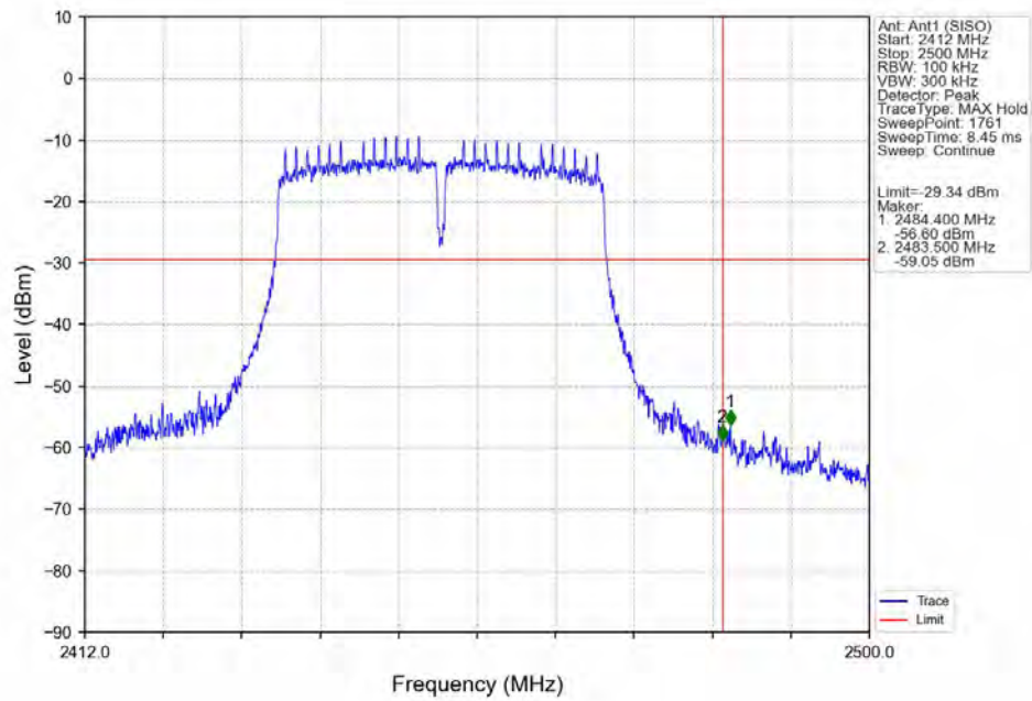
802.11ax(HEW40)_HCH_2452MHz_Ant1 (SISO)_NTNV
