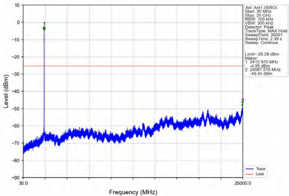
802.11ax(HEW20)_LCH_2412MHz_Ant1 (SISO)_NTNV
