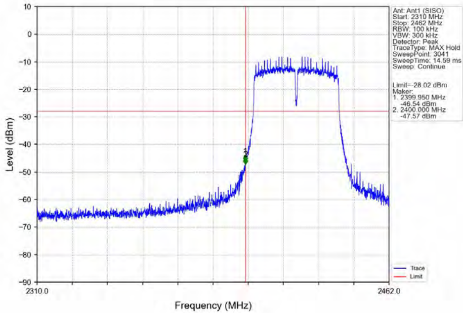
802.11ax(HEW40)_LCH_2422MHz_Ant1 (SISO)_NTNV
