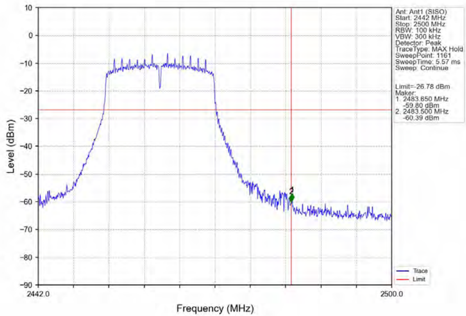
802.11ax(HEW20)_HCH_2462MHz_Ant1 (SISO)_NTNV
