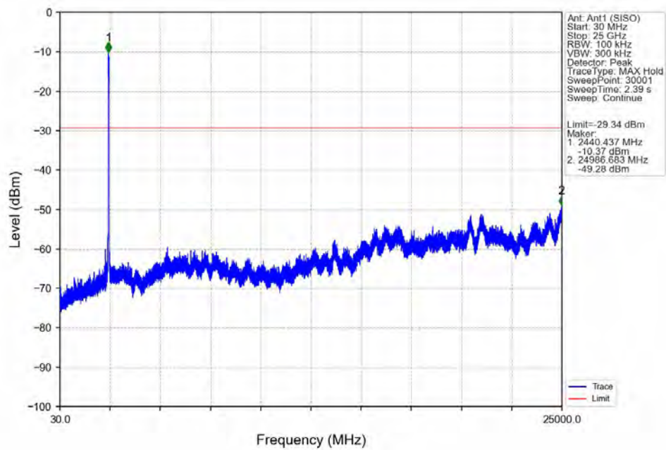
802.11ax(HEW40)_HCH_2452MHz_Ant1 (SISO)_NTNV
