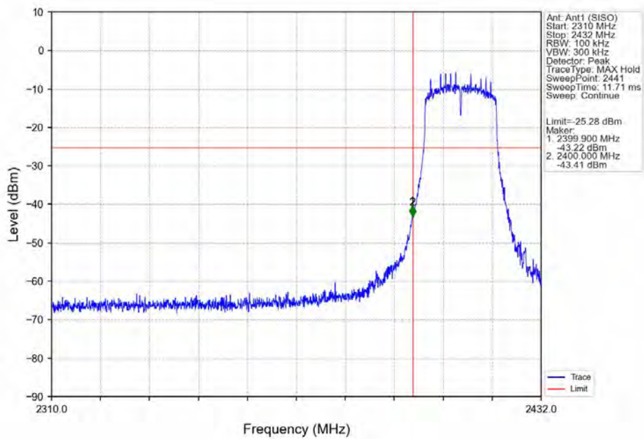
802.11ax(HEW20)_LCH_2412MHz_Ant1 (SISO)_NTNV
