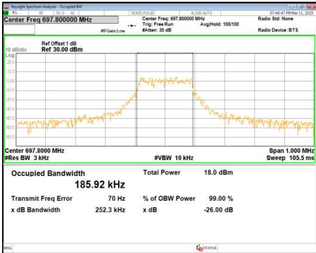
Band71 QPSK Channel=133470 nTones=1@0 Spacing=15kHz
