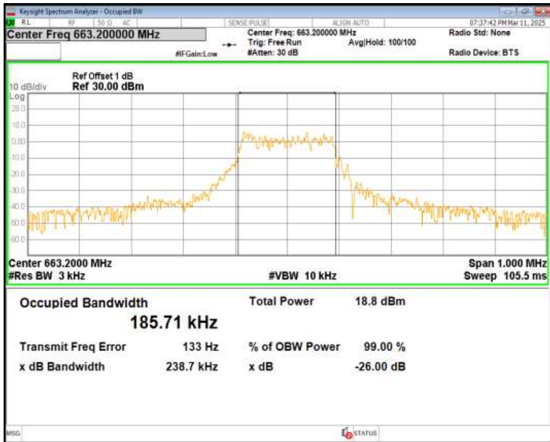
Band71 QPSK Channel=133124 nTones=1@0 Spacing=15kHz
