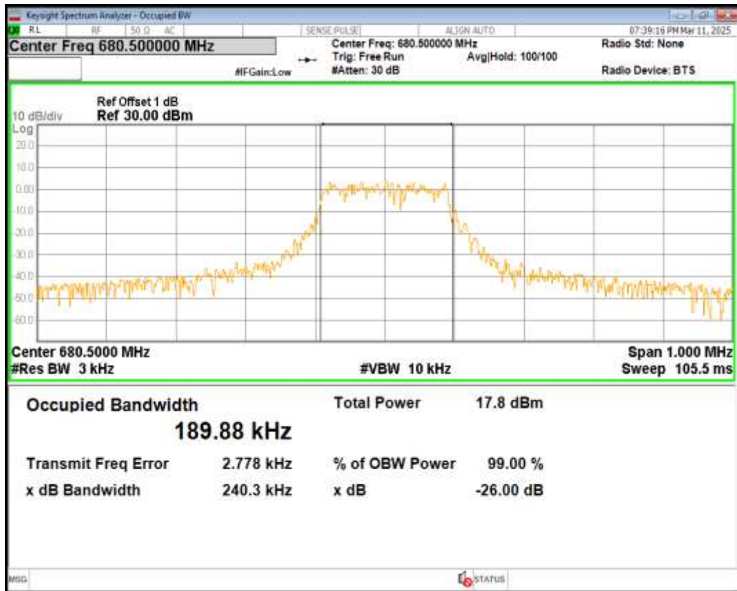
Band71 QPSK Channel=133297 nTones=1@0 Spacing=15kHz
