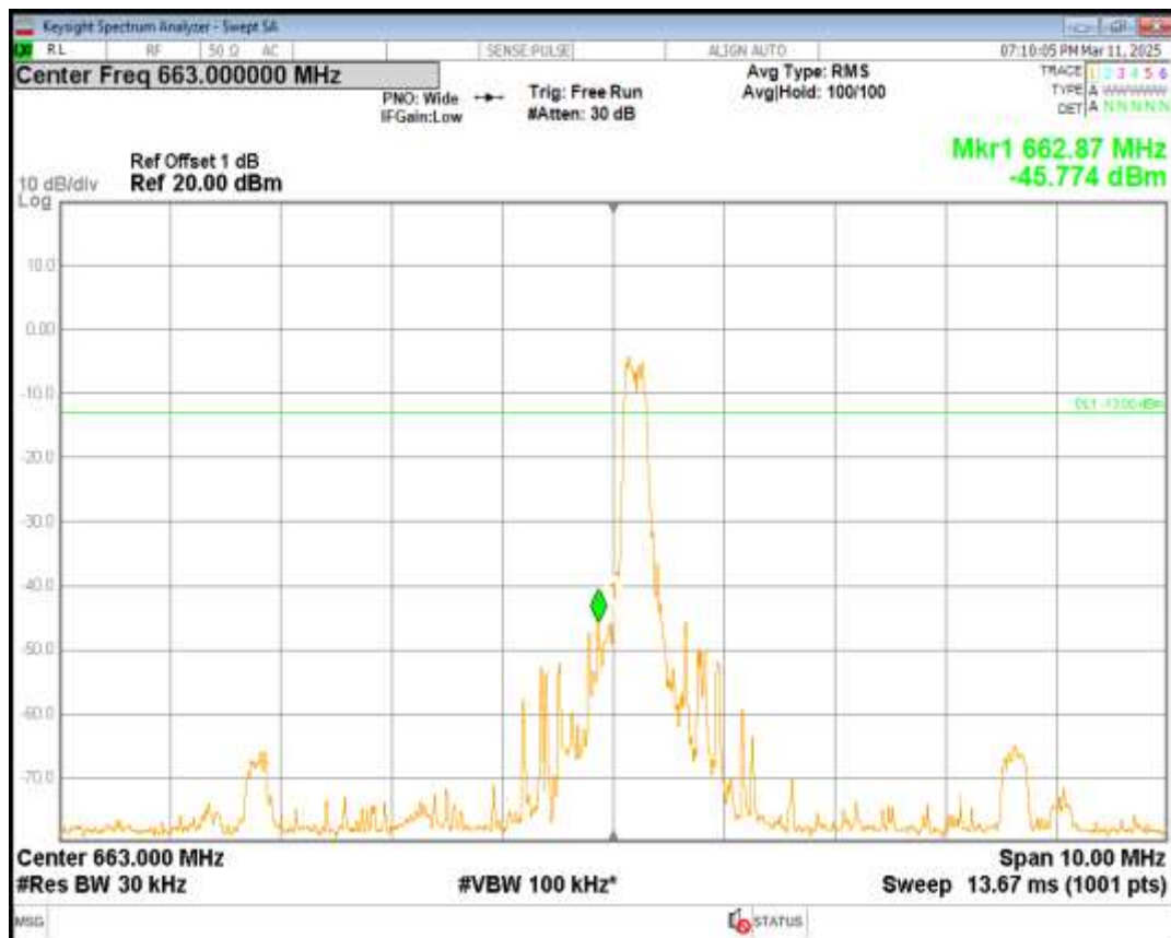
Band71 QPSK Channel=133124 nTones=1@0 Spacing=15kHz
