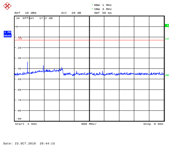
GSM 850 CH-High 1GHz ~ 9GHz
