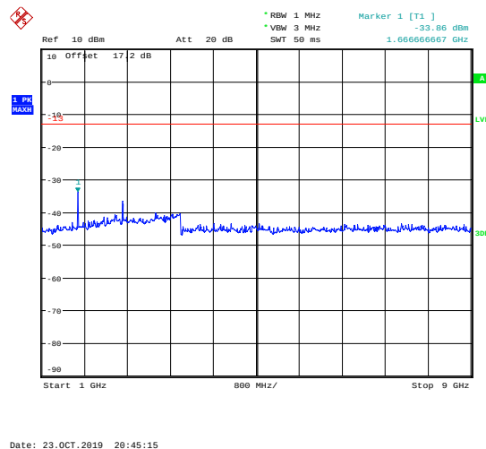
GSM 850 CH-High 1GHz ~ 9GHz
