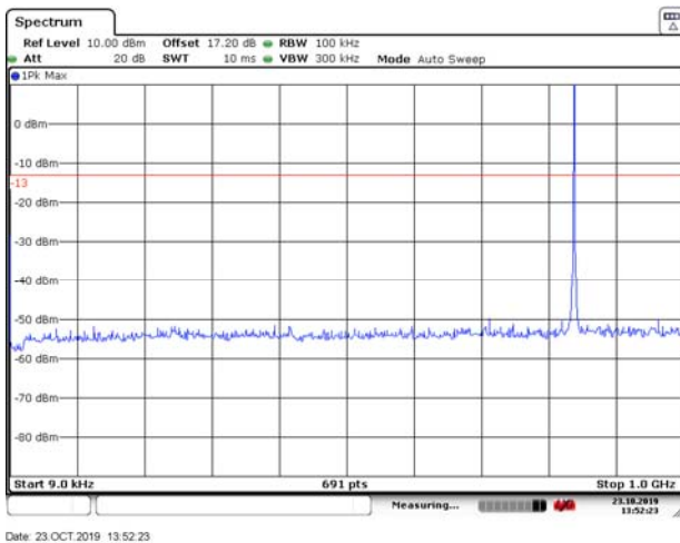
GSM 850 CH-Middle 9KHz ~ 1GHz
