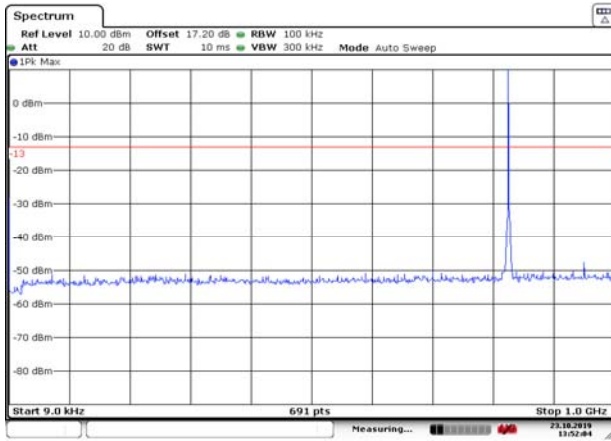
GSM 850 CH-Low 9KHz ~ 1GHz
