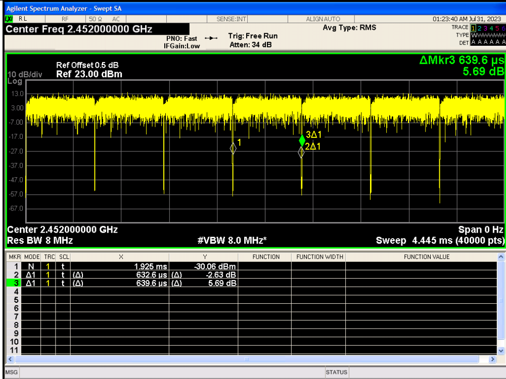
IEEE 802.11n_40MHz_Channel 9
