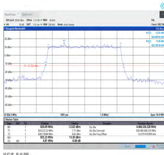
1-N5-PC3-15-5-L-4-DFT-64QAM-Outet_Full-25@0-A nt1-4.466-4.810-≤5-PASS
