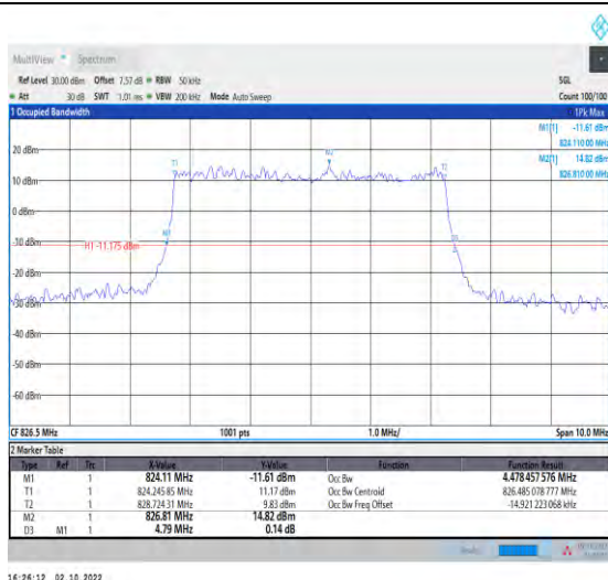
1-N5-PC3-15-5-L-1-DFT-QPSK-Outet_Full-25@0-An t1-4.478-4.790-≤5-PASS
