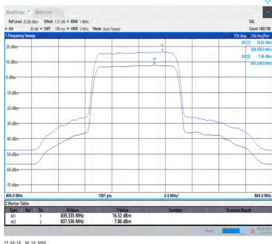
1-N5-PC3-15-20-L-1-DFT-256QAM-Outet_Full-100@ 0-Ant1-8.66-100%-0.00-8.66-PASS-≤13
