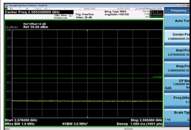
FDD07_20MHz_2510_Q16_fullIRB_ExtraBand s_Range_2576~2595
