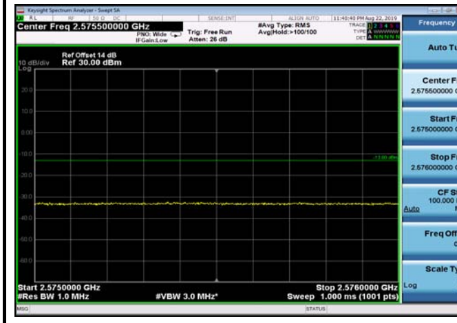
FDD07_20MHz_2560_QPSK_fullIRB_ExtraBan ds_Range_2575~2576
