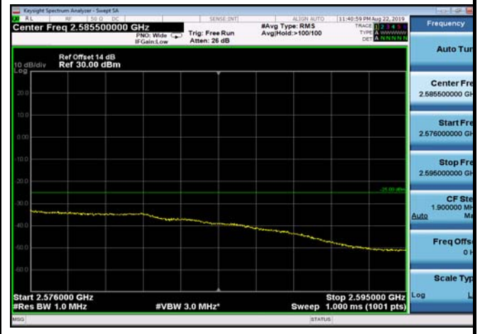
FDD07_20MHz_2560_QPSK_fullIRB_ExtraBan ds_Range_2576~2595
