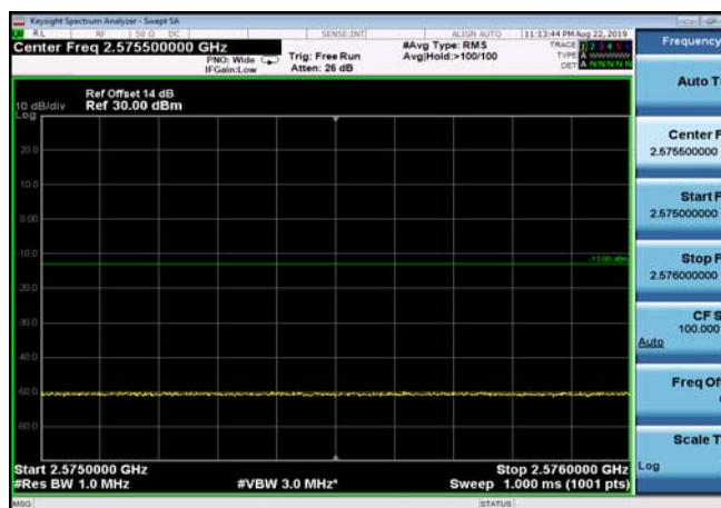
FDD07_20MHz_2510_Q16_fullIRB_ExtraBand s_Range_2575~2576
