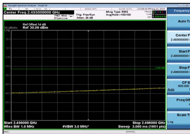
FDD07_10MHz_2505_Q16_fullRB_ExtraBand s_Range_2490~2496
