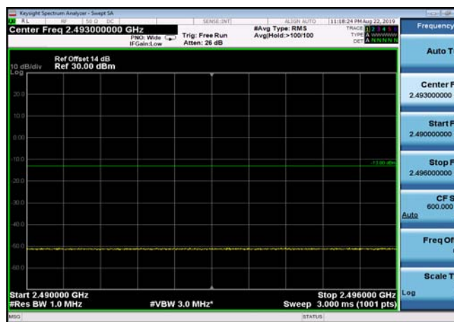
FDD07_5MHz_2567.5_QPSK_fullIRB_ExtraBa nds_Range_2490~2496
