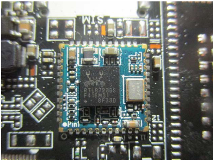
EUT –Wifi &BT Module View
