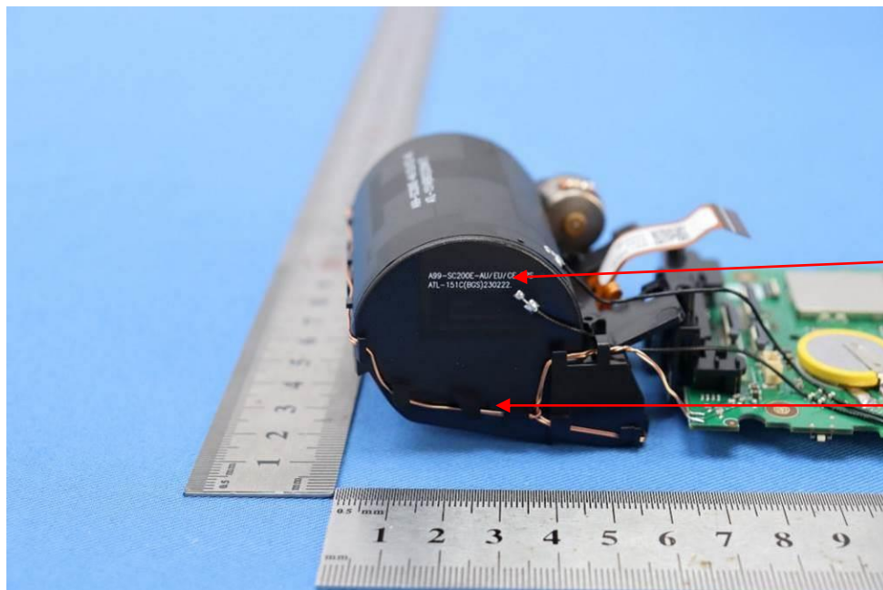
GPS(Rx) antenna
