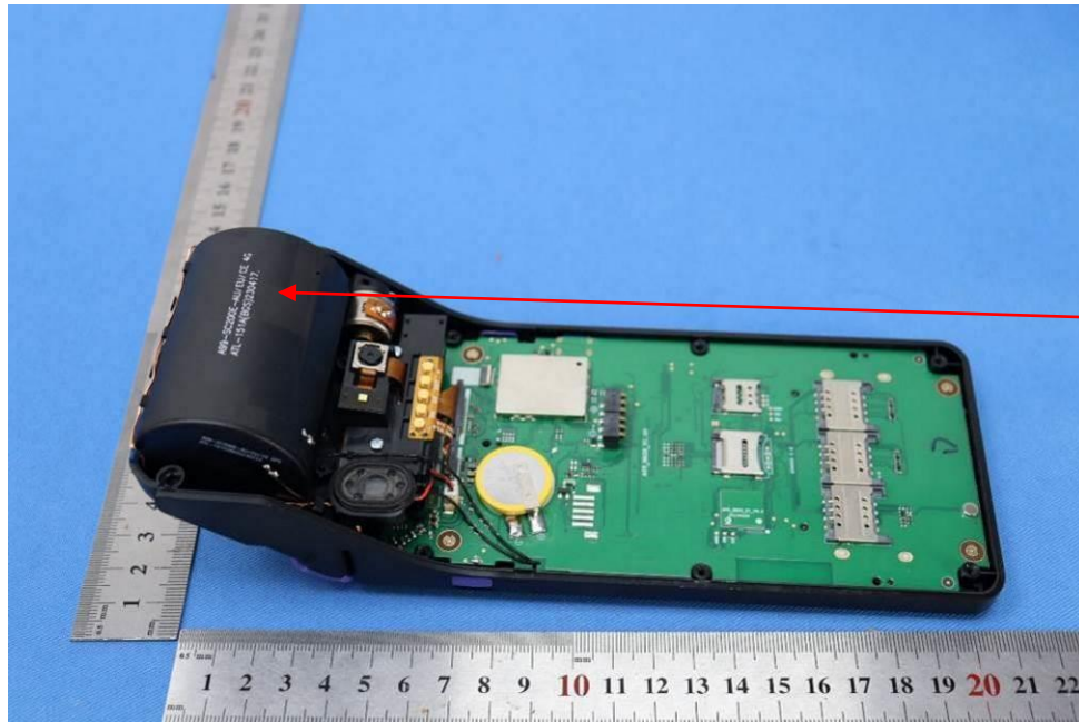
WWAN antenna
