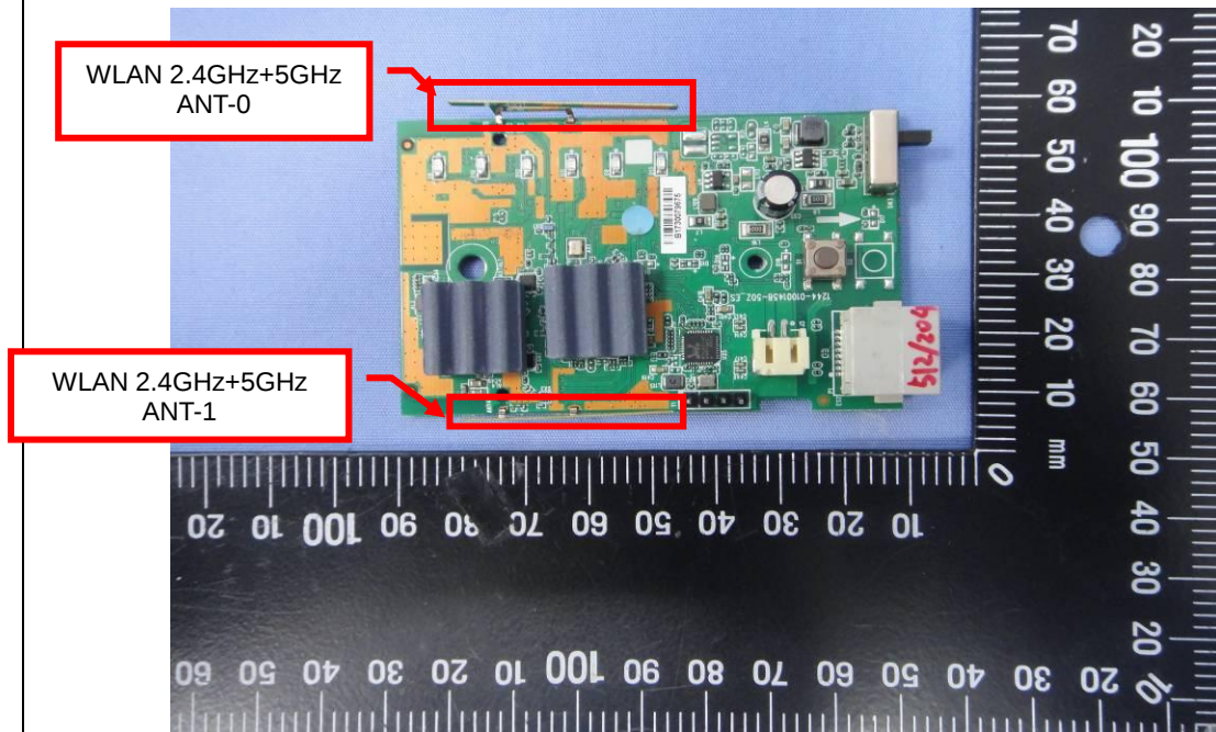
EUT Photo (2)
