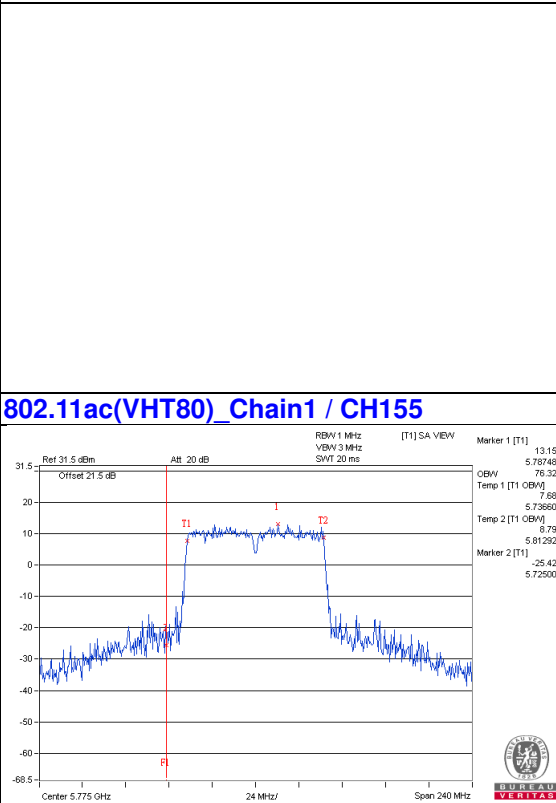
802.11ac(VHT80)_Chain1 / CH155
