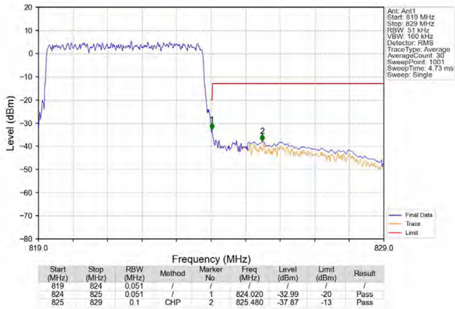
Band26a 5MHz 16QAM HCH 821.5MHz RB 25 0 NTN
