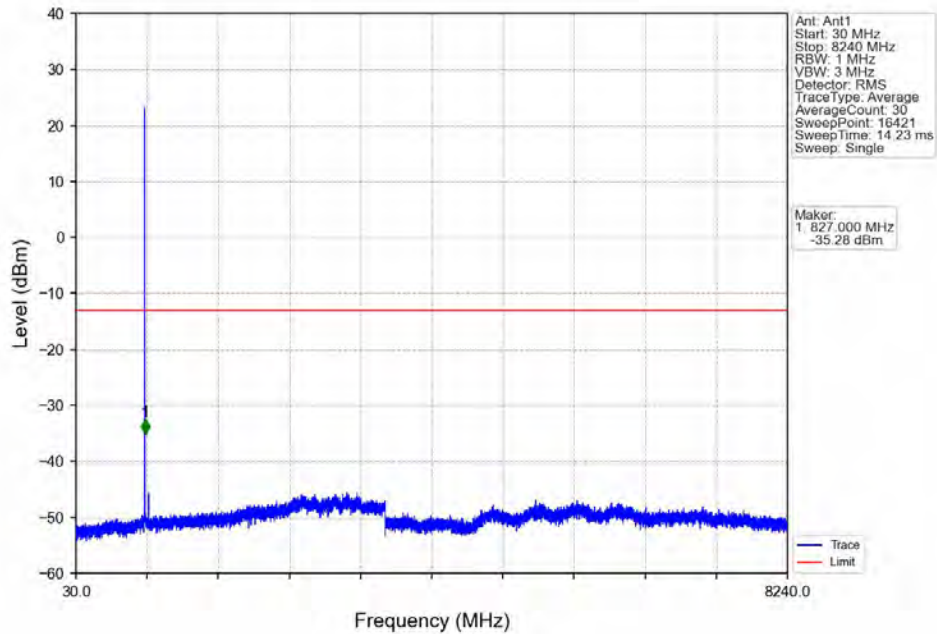
Band26a 1.4MHz QPSK HCH 823.3MHz RB 1 5 NTN
