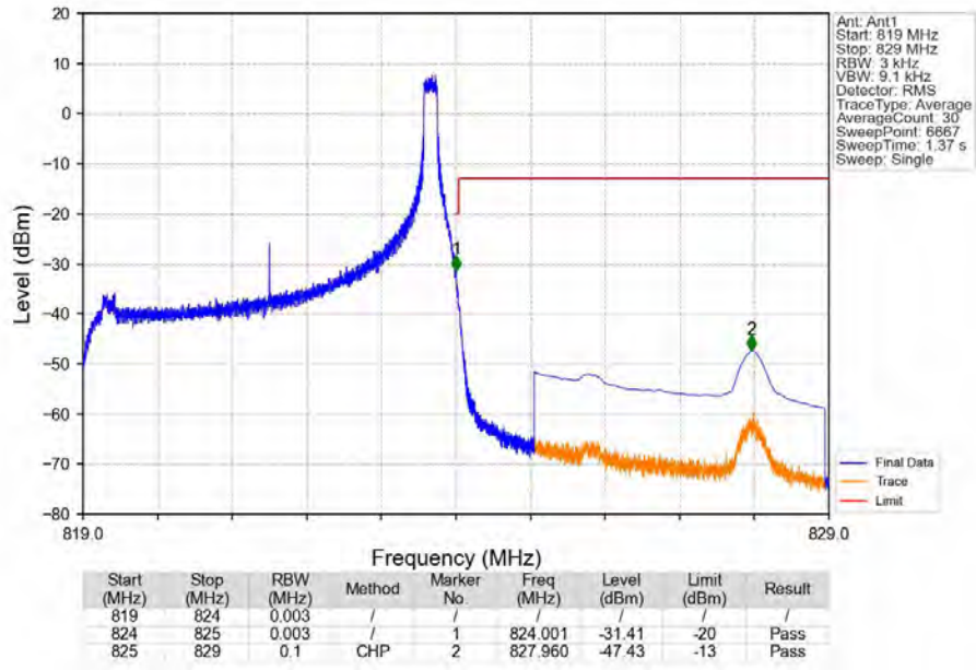
Band26a 5MHz 16QAM HCH 821.5MHz RB 1 24 NTN
