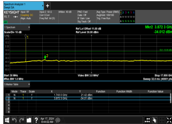
N66(5M)_CP- OFDM_QPSK_Edge_1RB_Left_Mid_CH
