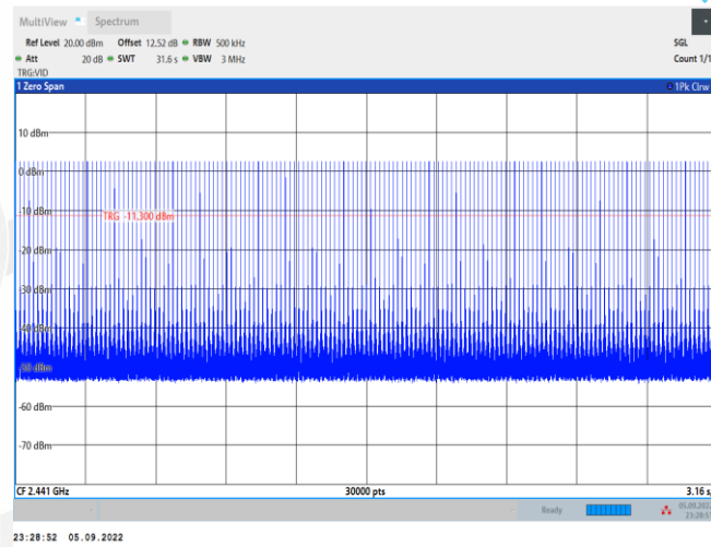
DH5_Ant1_Hop
