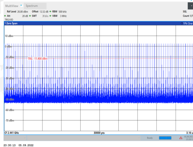
2DH1_Ant1_Hop
