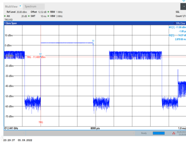
DH5_Ant1_Hop
