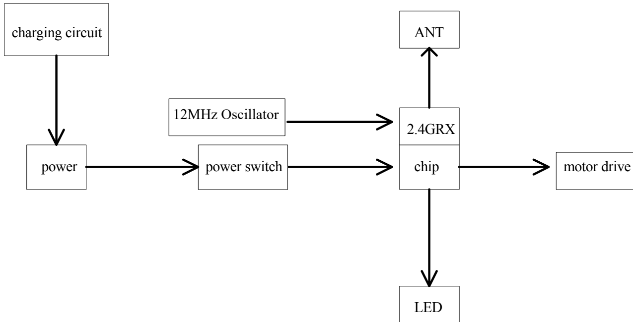
66804RXV13 block diagram
