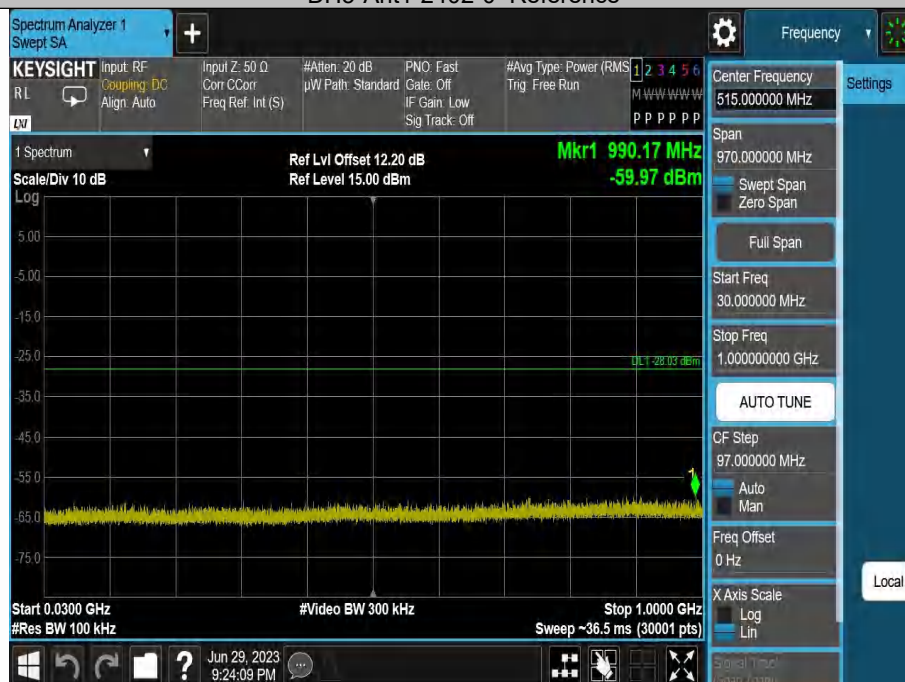
DH5-Ant1-2402-30~1000
