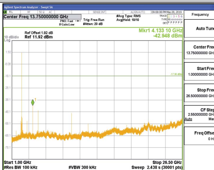
DH1_Ant1_2480_1000~26500
