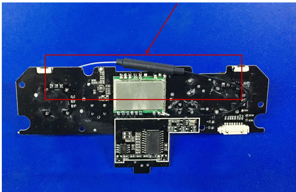
Antenna
