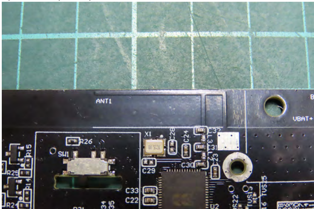
(10) EUT Photo (Antenna)
