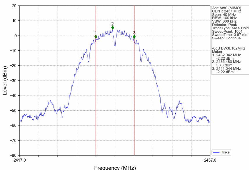
802.11b_MCH_2437MHz_Ant0 (MIMO)_NTNV
