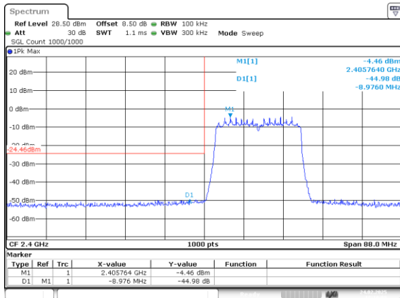
802.11ax20_2412MHz_Chain 1
