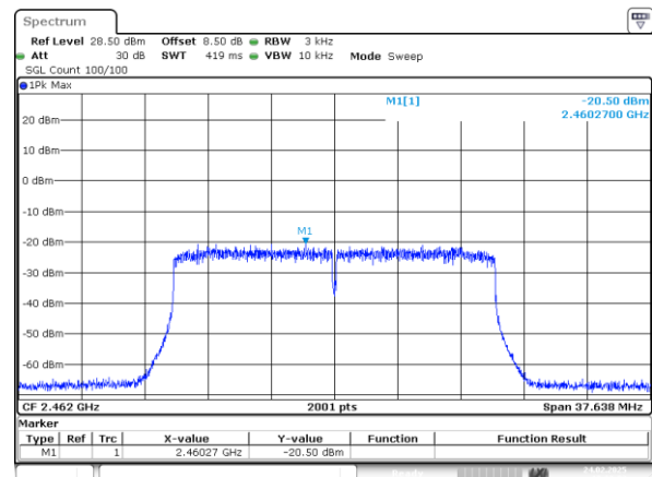
802.11ax20_2462MHz_Chain 1
