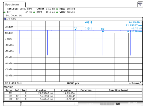
802.11b_2437MHz_Chain 1
