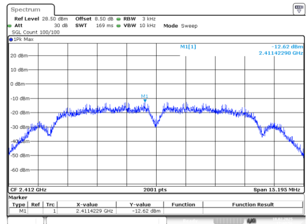
802.11b_2412MHz_Chain 1
