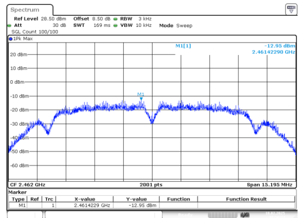
802.11b_2462MHz_Chain 1
