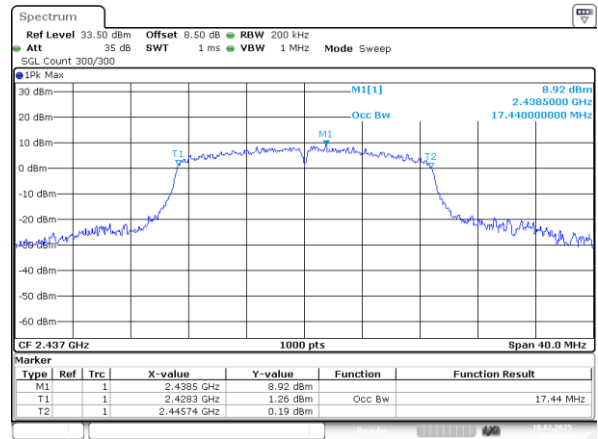
802.11n20_2437MHz_Chain 0
