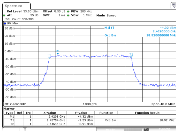
802.11ax20_2437MHz_Chain 1
