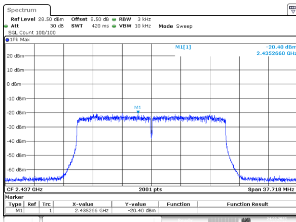
802.11ax20_2437MHz_Chain 1
