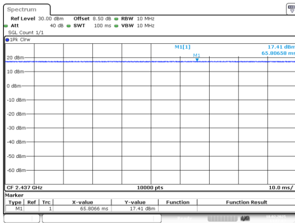
802.11b_2437MHz_Chain 0
