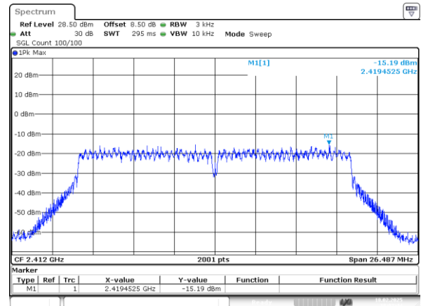
802.11n20_2412MHz_Chain 1
