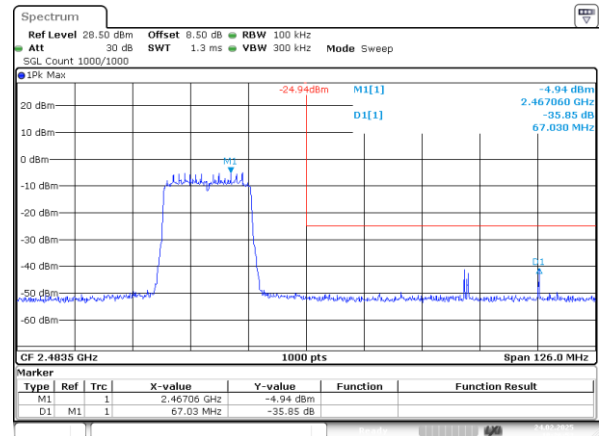
802.11ax20_2462MHz_Chain 1
