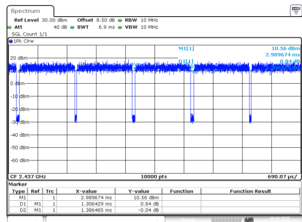
802.11n20_2437MHz_Chain 1
