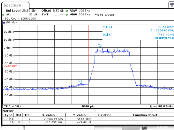
802.11n20_2412MHz_Chain 1
