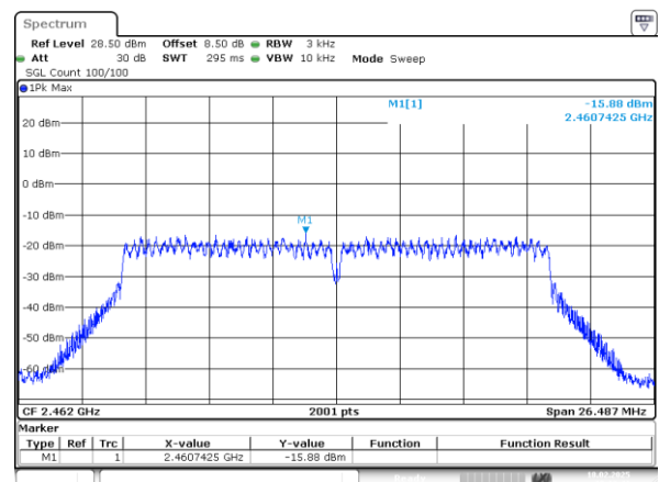
802.11n20_2462MHz_Chain 1
