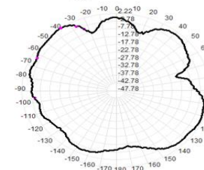
2400.0MHz Total(E1), Max= 2.22dBi
