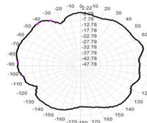
2400.0MHz Total(E2), Max= 1.02dBi
