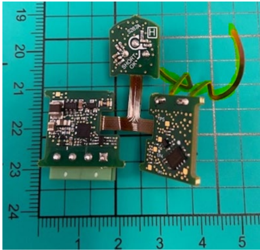
Internal Photos: (Antenna Highlighted)
