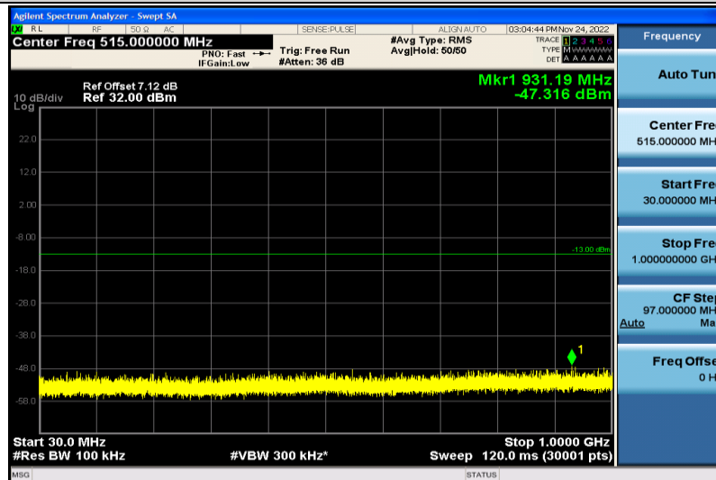
Band2-5MHz-QPSK-19175-1RB#0-30~1000MHz
