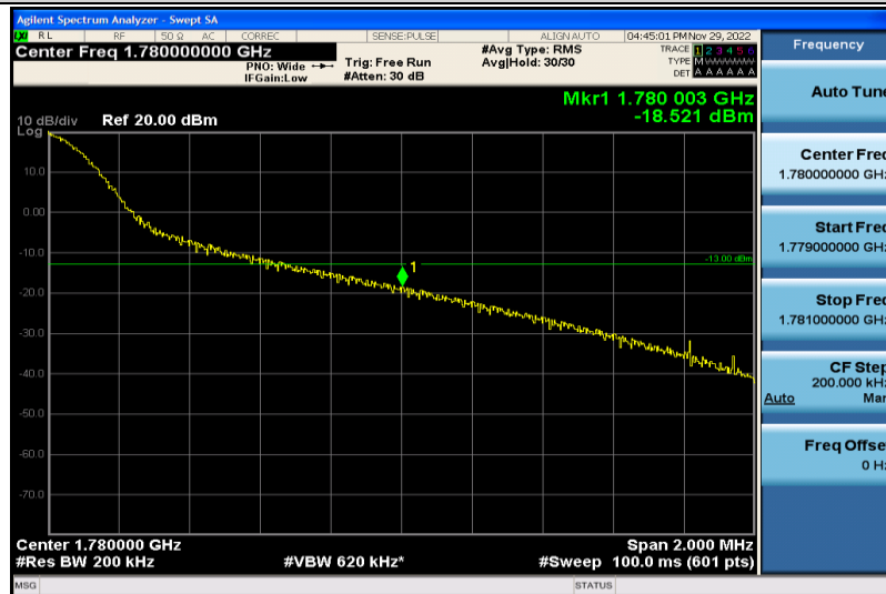
Band66-20MHz-QPSK-132572-1RB#99
