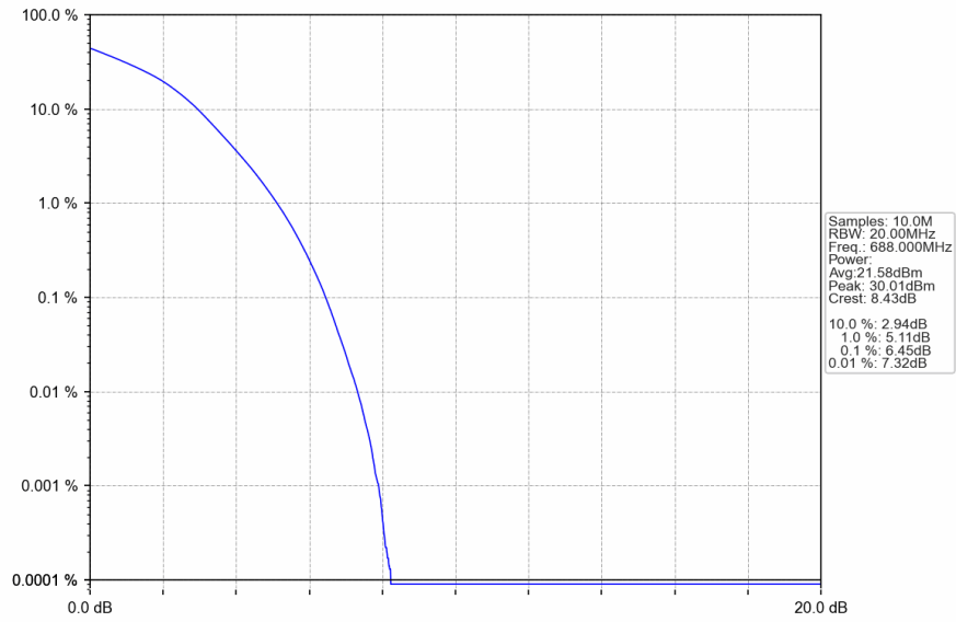
Band71_20MHz_16QAM_HCH_688MHz_RB_100_0_NTNV
