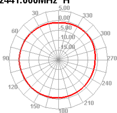
2441.000MHz H
