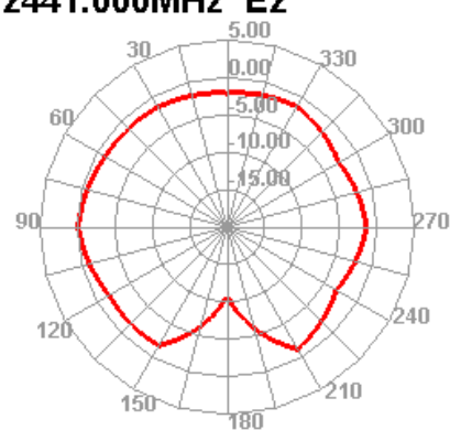
2441.000MHz E2
