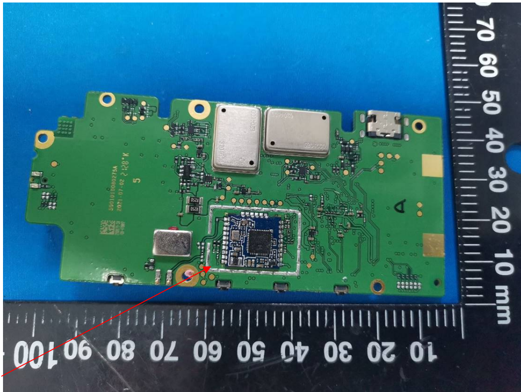
BT Module
