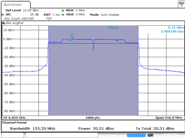
MIMO B-802.11ax/be-160MHz-Ch15-6025MHz-MCS0
