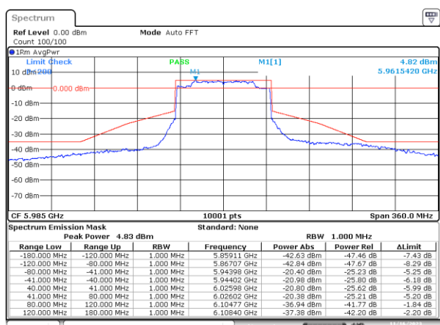
MIMO B-802.11ax/be-80MHz-Ch7-5985MHz-MCS0
