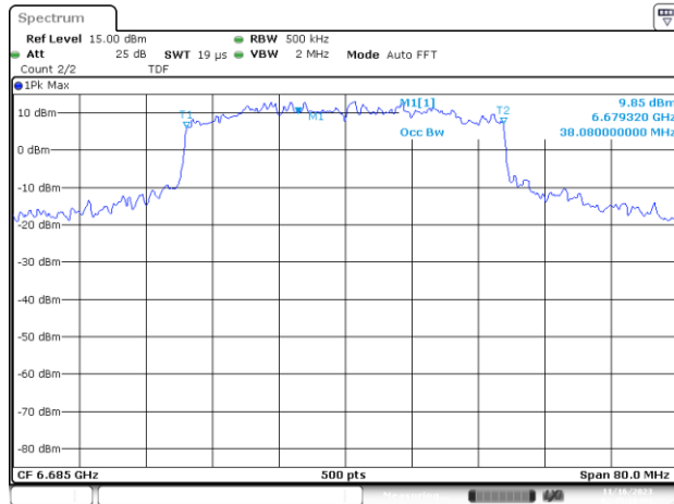
UNII7 SISO B 802.11ax/be40 ch147 6685MHz 99%
