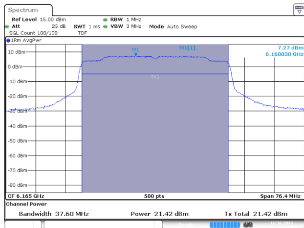
MIMO A-802.11ax/be-40MHz-Ch43-6165MHz-MCS0
