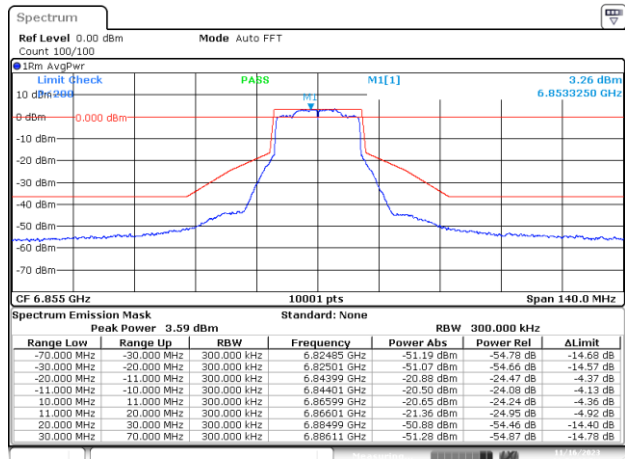
MIMO B-802.11ax/be-20MHz-Ch181-6855MHz-MCS0
