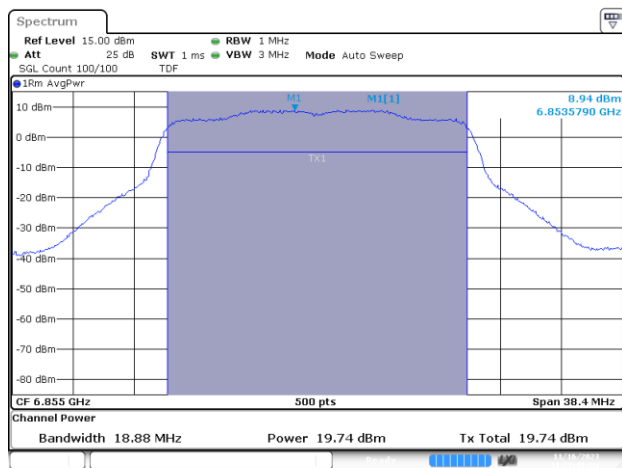
MIMO A-802.11ax/be-20MHz-Ch181-6855MHz-MCS0
