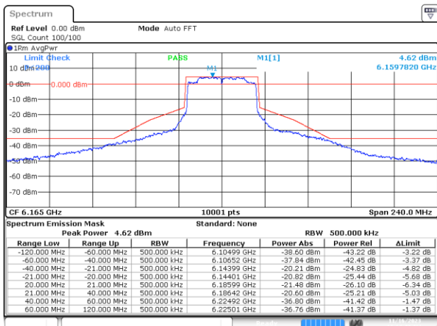
MIMO A-802.11ax/be-40MHz-Ch43-6165MHz-MCS0
