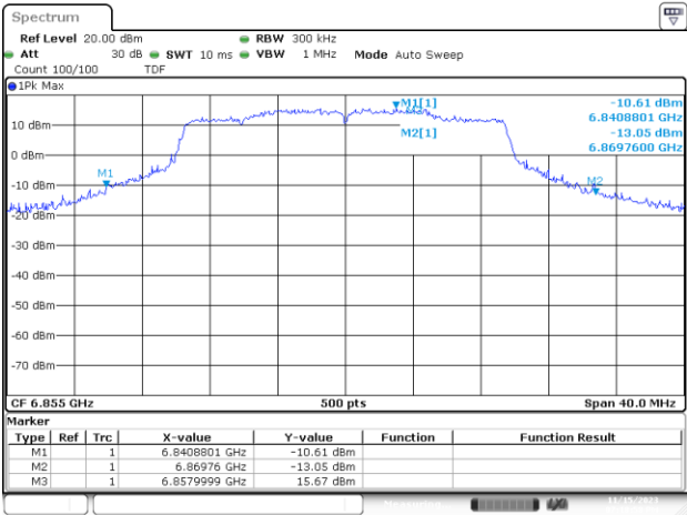
UNII7 SISO A 802.11ax/be20 ch181 6855MHz 26dB
