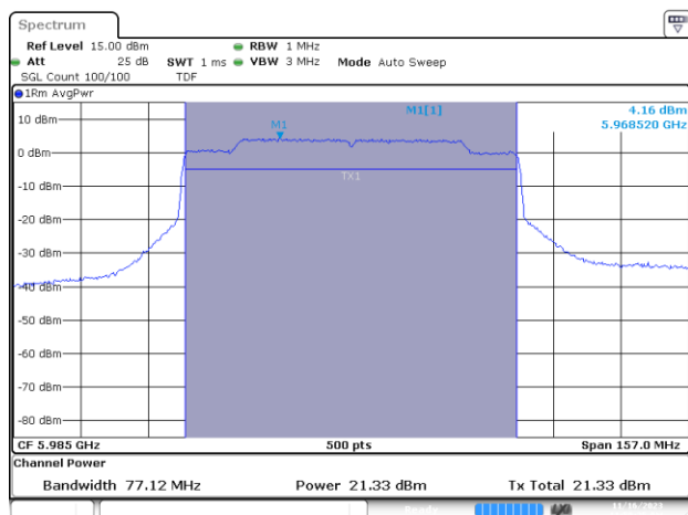
MIMO A-802.11ax/be-80MHz-Ch7-5985MHz-MCS0
