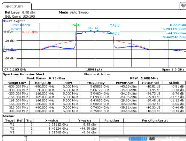
MIMO A-802.11be-320MHz-Ch63-6265MHz-MCS0
