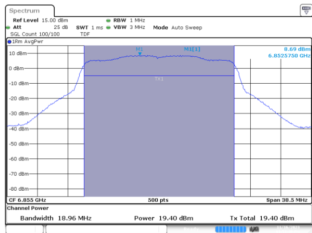
MIMO B-802.11ax/be-20MHz-Ch181-6855MHz-MCS0
