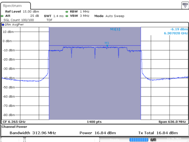
MIMO A-802.11be-320MHz-Ch63-6265MHz-MCS0
