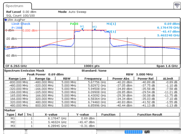
MIMO B-802.11be-320MHz-Ch63-6265MHz-MCS0
