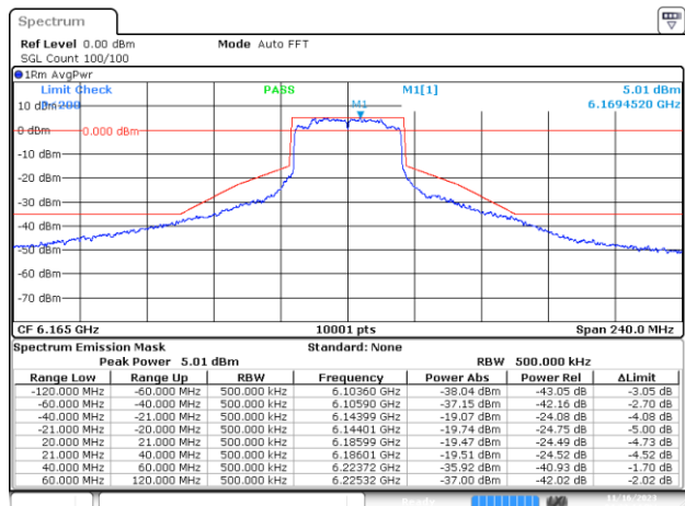
MIMO B-802.11ax/be-40MHz-Ch43-6165MHz-MCS0
