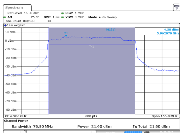
MIMO B-802.11ax/be-80MHz-Ch7-5985MHz-MCS0
