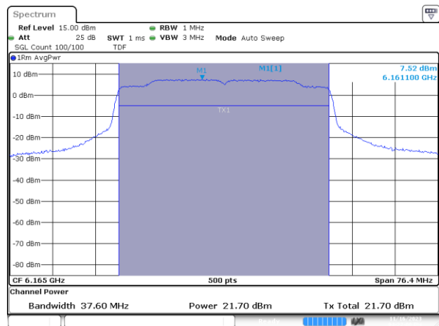
MIMO B-802.11ax/be-40MHz-Ch43-6165MHz-MCS0
