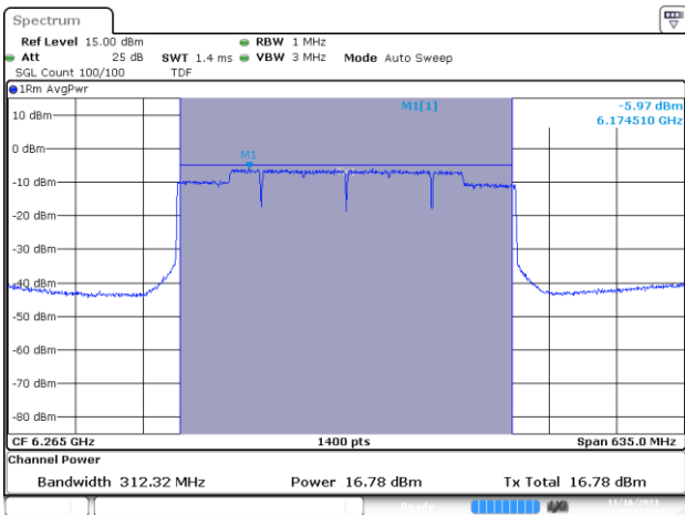
MIMO B-802.11be-320MHz-Ch63-6265MHz-MCS0
