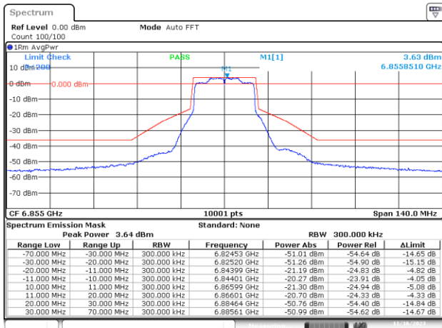
MIMO A-802.11ax/be-20MHz-Ch181-6855MHz-MCS0
