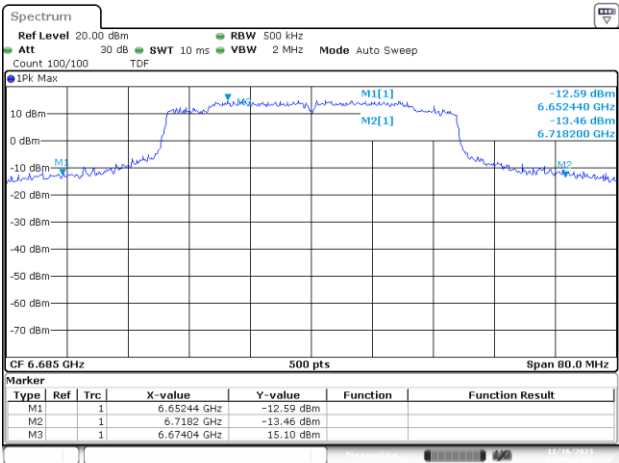
UNII7 SISO B 802.11ax/be40 ch147 6685MHz 26dB
