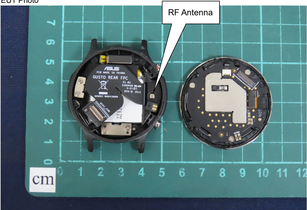
(9) EUT Photo
