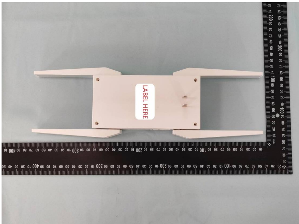
(6) EUT Photo
