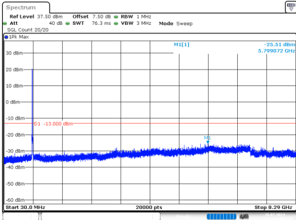
10MHz_Low_QPSK_50@0 -25.51dBm
