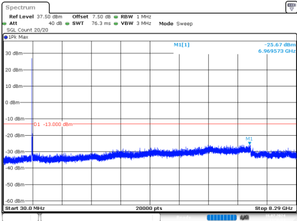
10MHz_Low_QPSK_1@0 -25.67dBm
