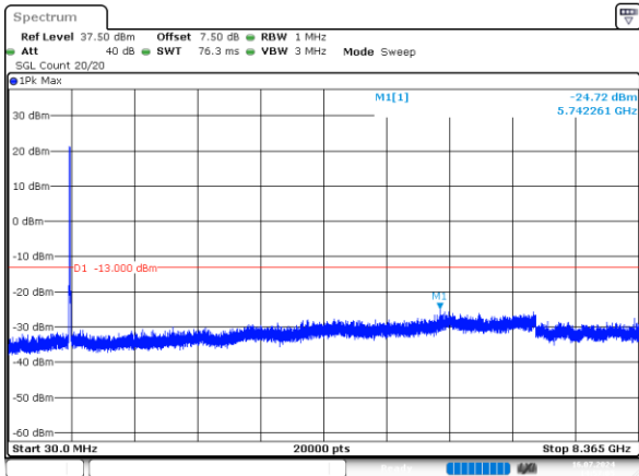
10MHz_Middle_QPSK_50@0 -24.72dBm
