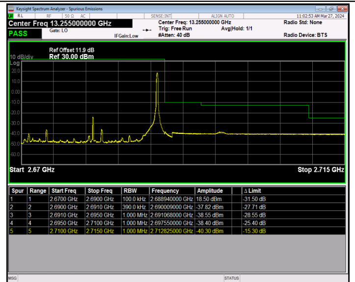
Band41_20MHz_QPSK_41490_1RB#99
