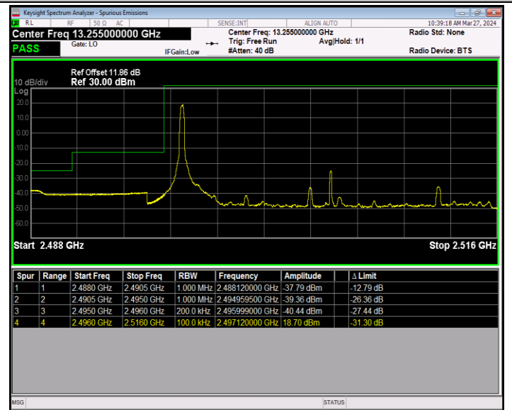
Band41_20MHz_QPSK_39750_1RB#0
