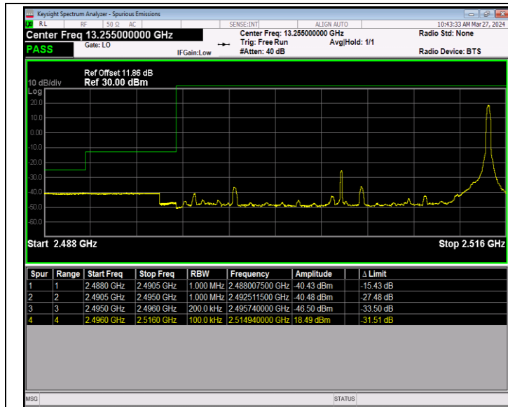
Band41_20MHz_QPSK_39750_1RB#99
