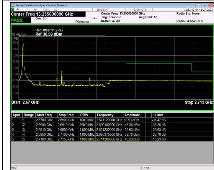
Band41_20MHz_QPSK_41490_1RB#0
