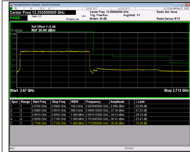
Band41_20MHz_QPSK_41490_100RB#0
