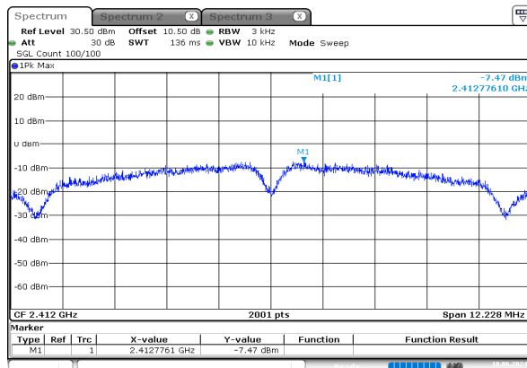
b_2412MHz_Chain 0
