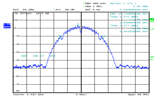
b_2437MHz_Chain 0
