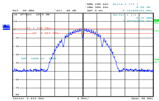
b_2412MHz_Chain 0
