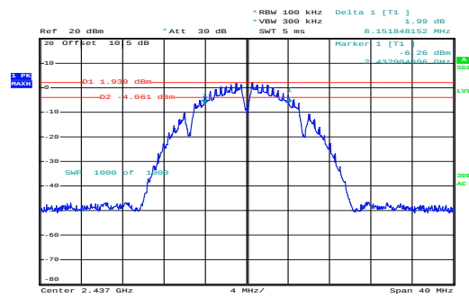
b_2437MHz_Chain 0
