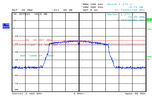
n20_2462MHz_Chain 0
