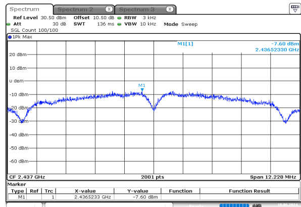
b_2437MHz_Chain 0
