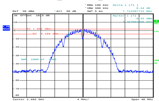
b_2462MHz_Chain 0
