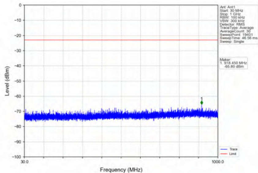
n41_30kHz_SISO_NTNV_60MHz_DFT-s-OFDM QPSK_2659.98MHz_Inner_1RB_Right
