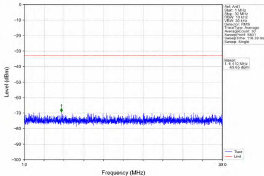
n41_30kHz_SISO_NTNV_90MHz_CP-OFDM_QPSK_2541MHz_Edge_1RB_Left
