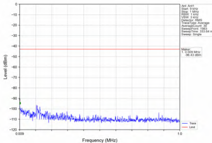
n41_30kHz_SISO_NTNV_60MHz_DFT-s-OFDM_PI/2_BPSK_2526MHz_Inner_1RB_Left
