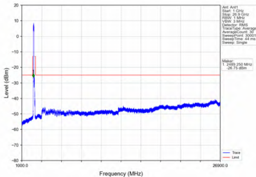
n41_30kHz_SISO_NTNV_90MHz_DFT-s-OFDM QPSK_2541MHz_Inner_1RB_Left
