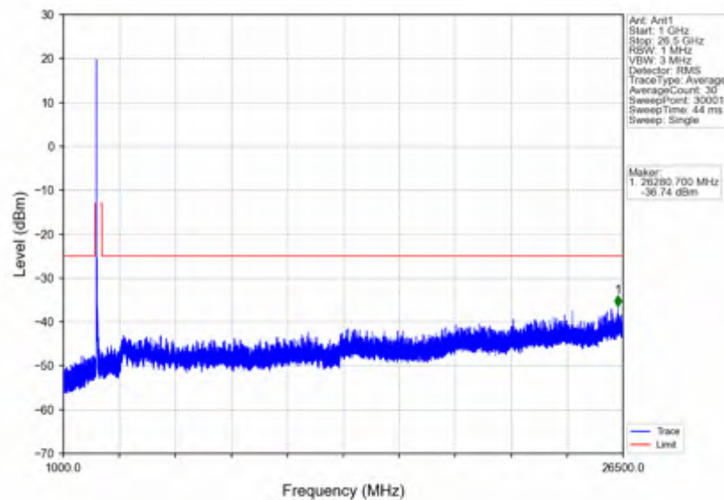
n41_30kHz_SISO_NTNV_60MHz_DFT-s-OFDM QPSK_2526MHz_Edge_1RB_Left
