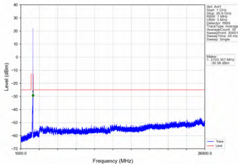
n41_30kHz_SISO_NTNV_60MHz_DFT-s-OFDM QPSK_2659.98MHz_Inner_1RB_Right
