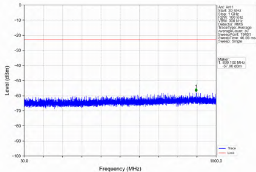
n41_30kHz_SISO_NTNV_90MHz_DFT-s-OFDM QPSK_2541MHz_Edge_1RB_Left
