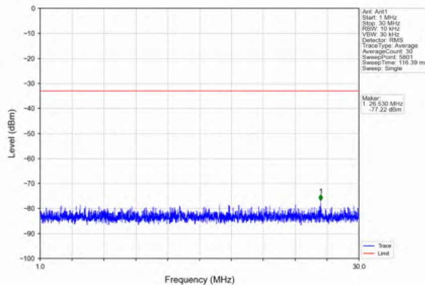
n41_30kHz_SISO_NTNV_60MHz_CP-OFDM_QPSK_2526MHz_Inner_1RB_Left
