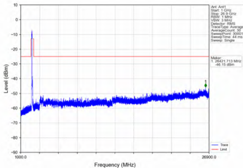
n41_30kHz_SISO_NTNV_80MHz_DFT-s-OFDM QPSK_2536.02MHz_Inner_1RB_Left
