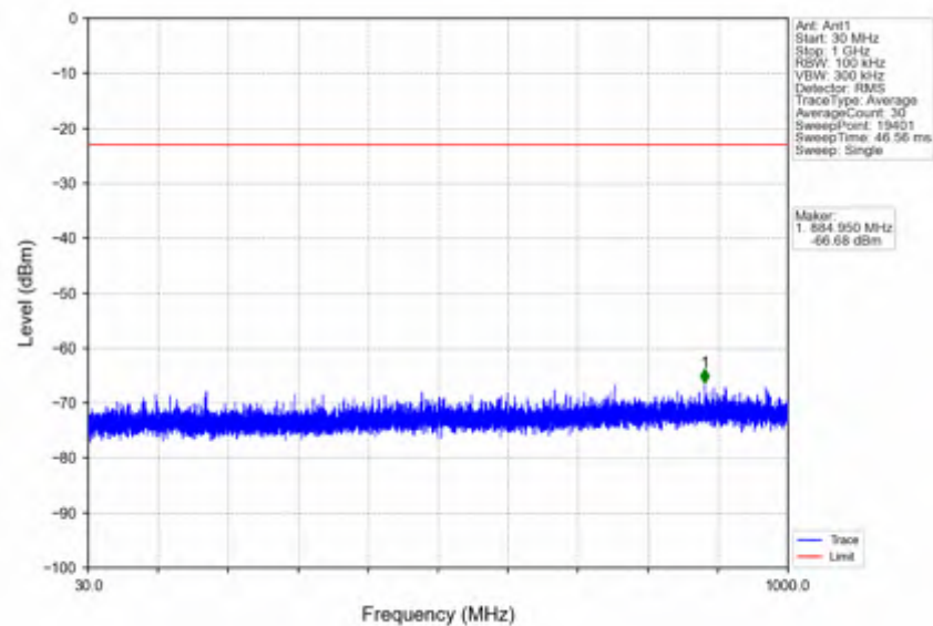
n41_30kHz_SISO_NTNV_60MHz_DFT-s-OFDM QPSK_2526MHz_Inner_1RB_Left
