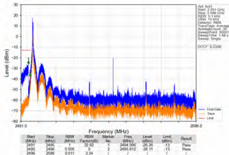
n41_30kHz_SISO_NTNV_90MHz_DFT-s-OFDM_PI/2_BPSK_2541MHz_Inner_1RB_Left
