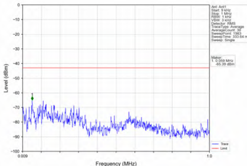
n41_30kHz_SISO_NTNV_90MHz_DFT-s-OFDM_PI/2_BPSK_2541MHz_Inner_1RB_Left
