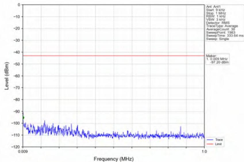
n41_30kHz_SISO_NTNV_60MHz_DFT-s-OFDM QPSK_2659.98MHz_Inner_1RB_Right
