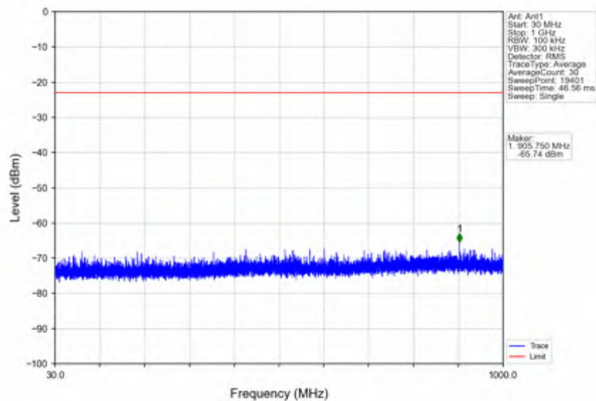
n41_30kHz_SISO_NTNV_60MHz_CP-OFDM QPSK_2659.98MHz_Inner_1RB_Right
