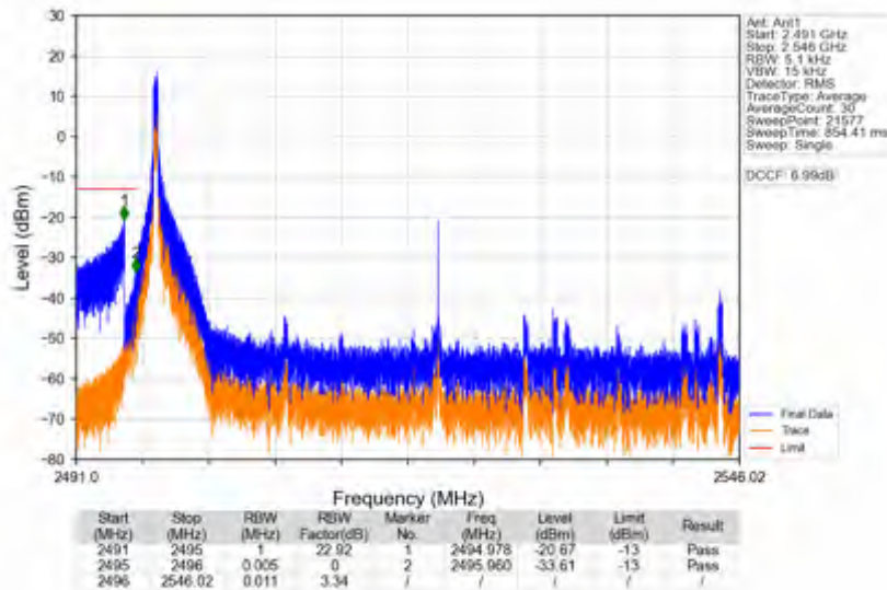
n41_30kHz_SISO_NTNV_50MHz_DFT-s-OFDM QPSK_2521.02MHz_Inner_1RB_Left
