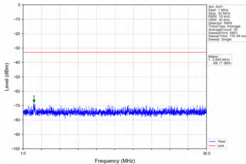
n41_30kHz_SISO_NTNV_60MHz_DFT-s-OFDM QPSK_2592.99MHz_Edge_1RB_Left
