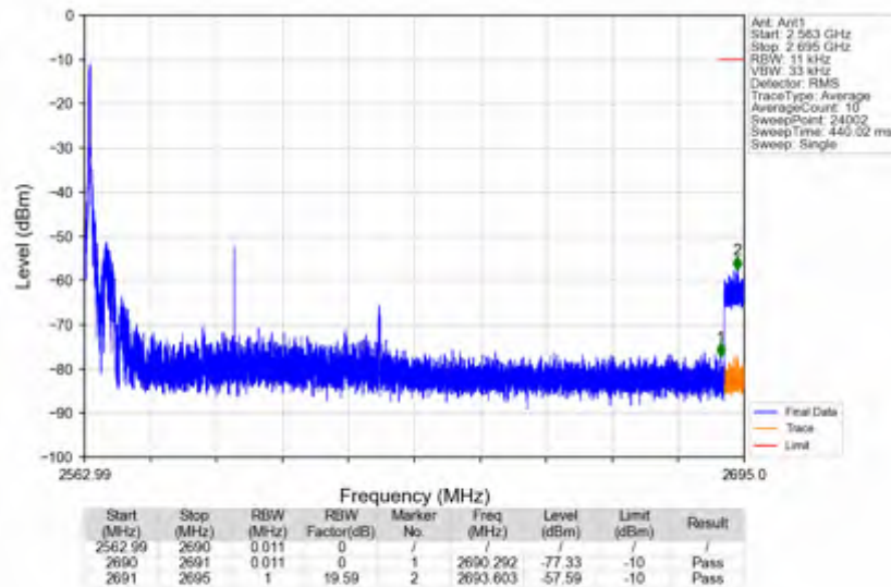
n41_30kHz_SISO_NTNV_60MHz_CP-OFDM QPSK_2592.99MHz_Edge_1RB_Left
