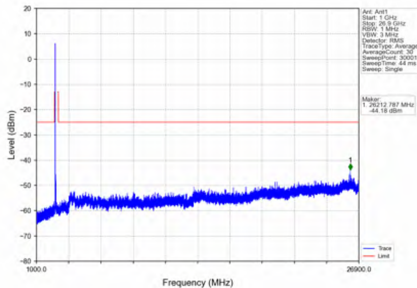
n41_30kHz_SISO_NTNV_60MHz_DFT-s-OFDM QPSK_2526MHz_Inner_1RB_Left
