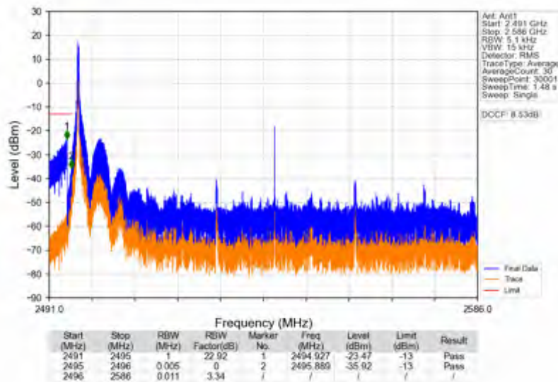
n41_30kHz_SISO_NTNV_90MHz_DFT-s-OFDM QPSK_2541MHz_Inner_1RB_Left
