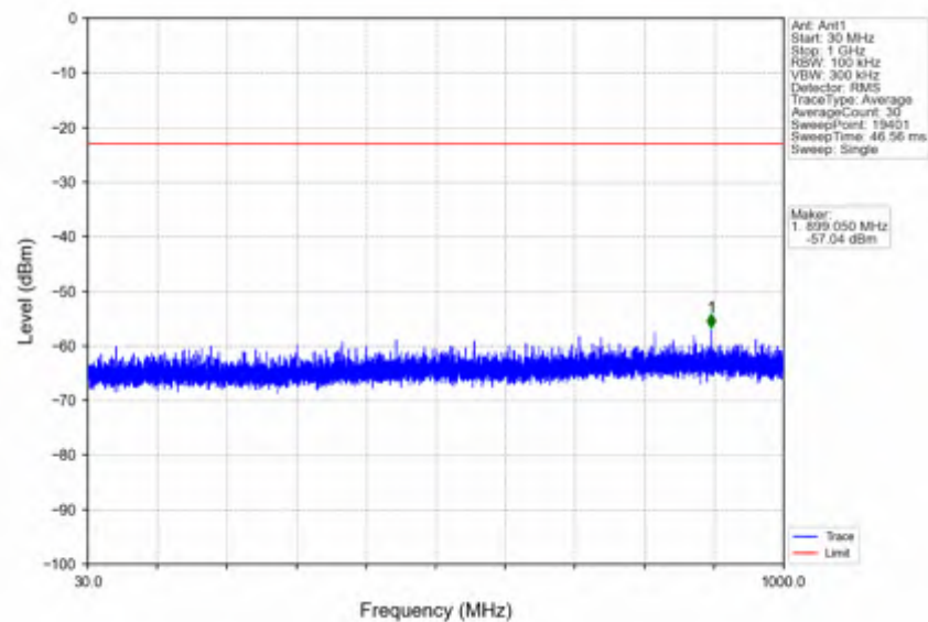
n41_30kHz_SISO_NTNV_60MHz_CP-OFDM_QPSK_2592.99MHz_Edge_1RB_Left
