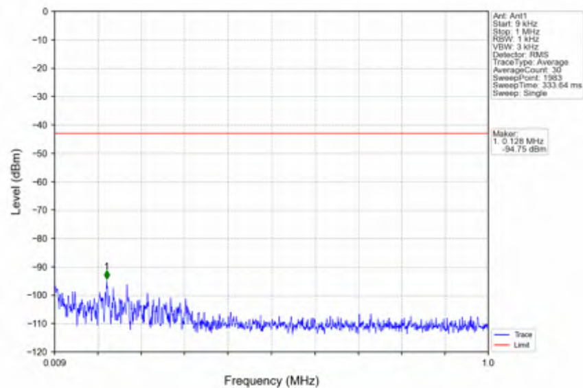
n41_30kHz_SISO_NTNV_60MHz_DFT-s-OFDM QPSK_2526MHz_Inner_1RB_Left
