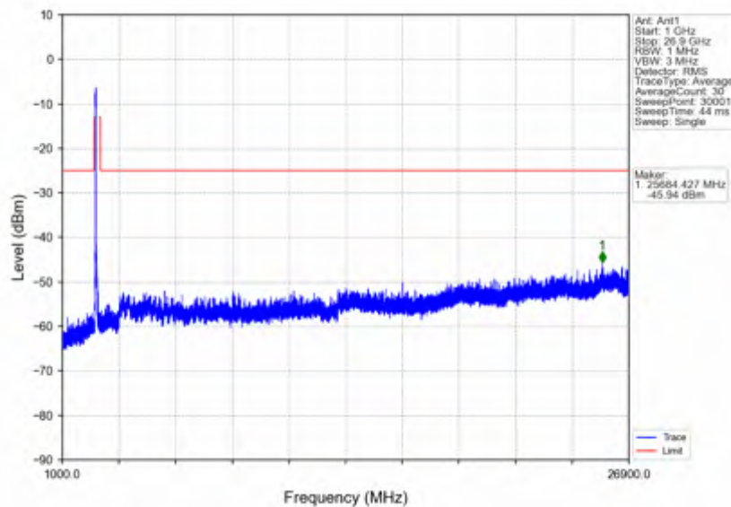
n41_30kHz_SISO_NTNV_50MHz_DFT-s-OFDM QPSK_2521.02MHz_Inner_1RB_Left
