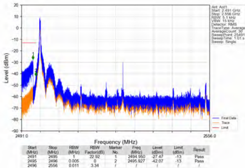
n41_30kHz_SISO_NTNV_60MHz_DFT-s-OFDM QPSK_2526MHz_Inner_1RB_Left
