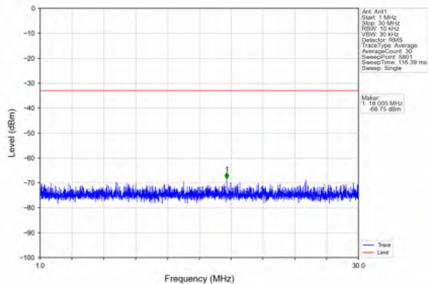
n41_30kHz_SISO_NTNV_90MHz_DFT-s-OFDM QPSK_2541MHz_Edge_1RB_Left
