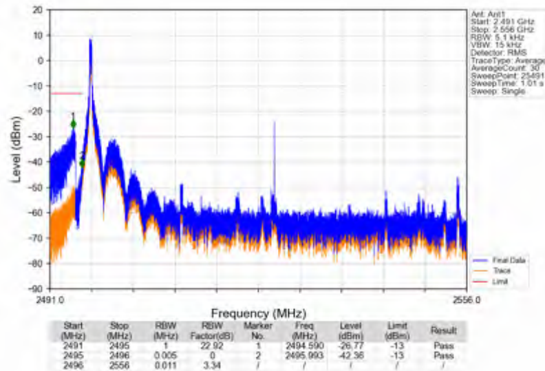
n41_30kHz_SISO_NTNV_60MHz_DFT-s-OFDM_PI/2_BPSK_2526MHz_Inner_1RB_Left
