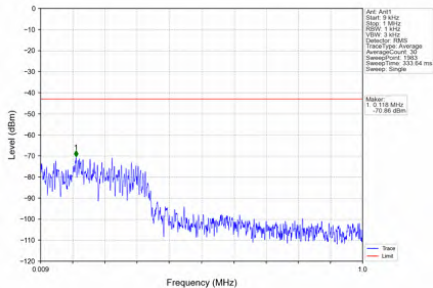
n41_30kHz_SISO_NTNV_60MHz_DFT-s-OFDM QPSK_2526MHz_Edge_1RB_Left
