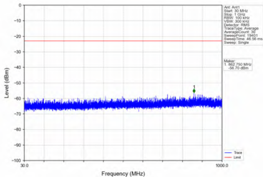
n41_30kHz_SISO_NTNV_60MHz_CP-OFDM_QPSK_2526MHz_Edge_1RB_Left
