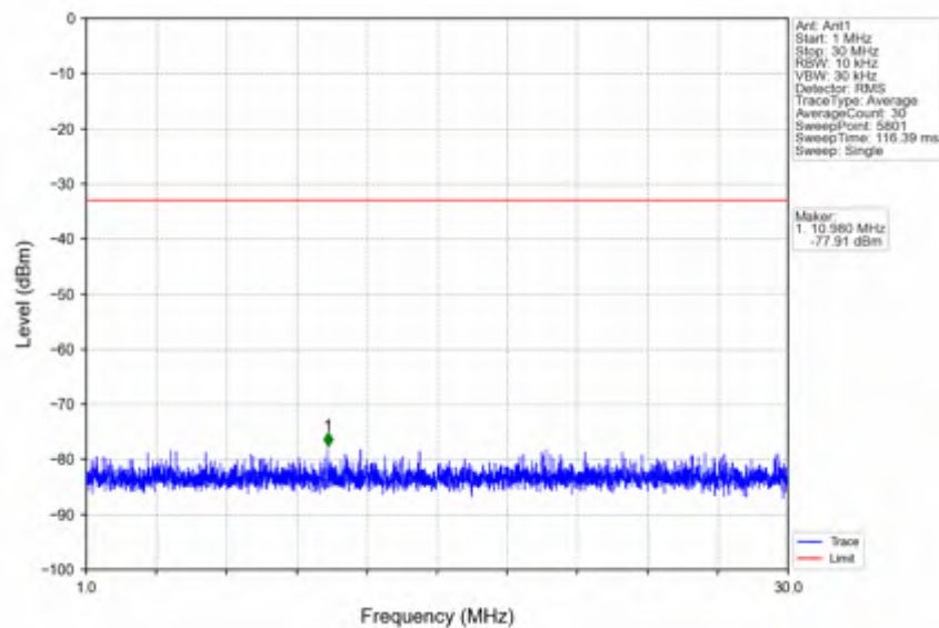
n41_30kHz_SISO_NTNV_60MHz_CP-OFDM QPSK_2659.98MHz_Inner_1RB_Right
