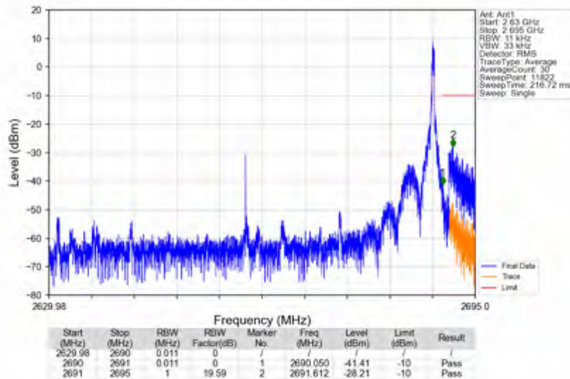
n41_30kHz_SISO_NTNV_60MHz_DFT-s-OFDM QPSK_2659.98MHz_Inner_1RB_Right
