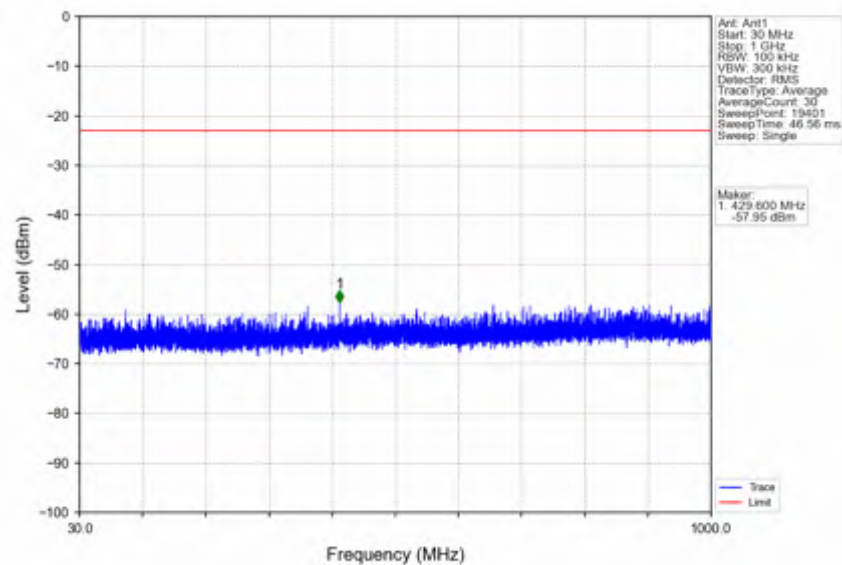
n41_30kHz_SISO_NTNV_60MHz_DFT-s-OFDM QPSK_2526MHz_Edge_1RB_Left
