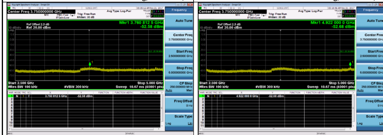
Case 4 2500MHz~5000MHz: 802.11n(40MHz),2422MHz,
