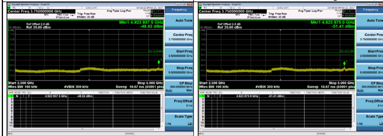
Case 42500MHz~5000MHz: 802.11g,2437MHz,
