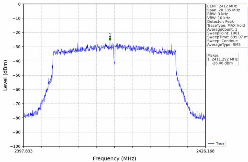
802.11ax(HEW20)_LCH_2412MHz_RU242_Left_Ant1 (SISO)_NTNV
