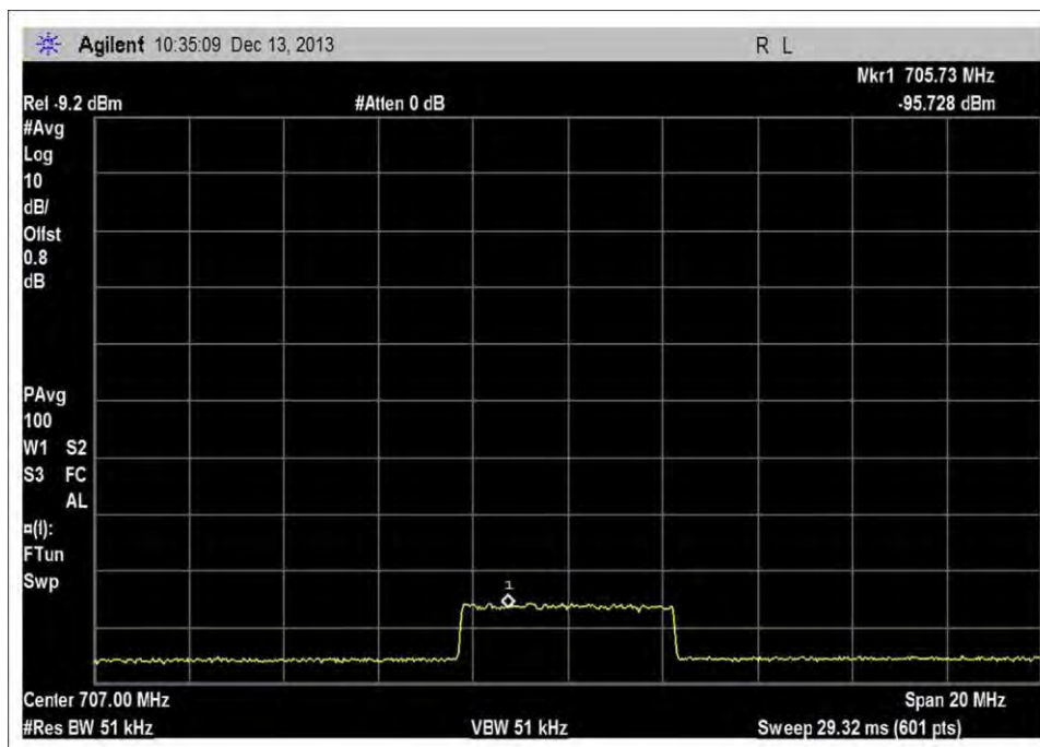
UL_698-716MHz_Input
