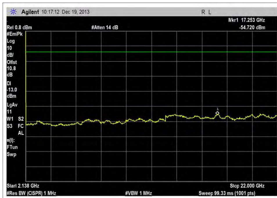
DL_2110-2155MHz_M_10LTE_2
