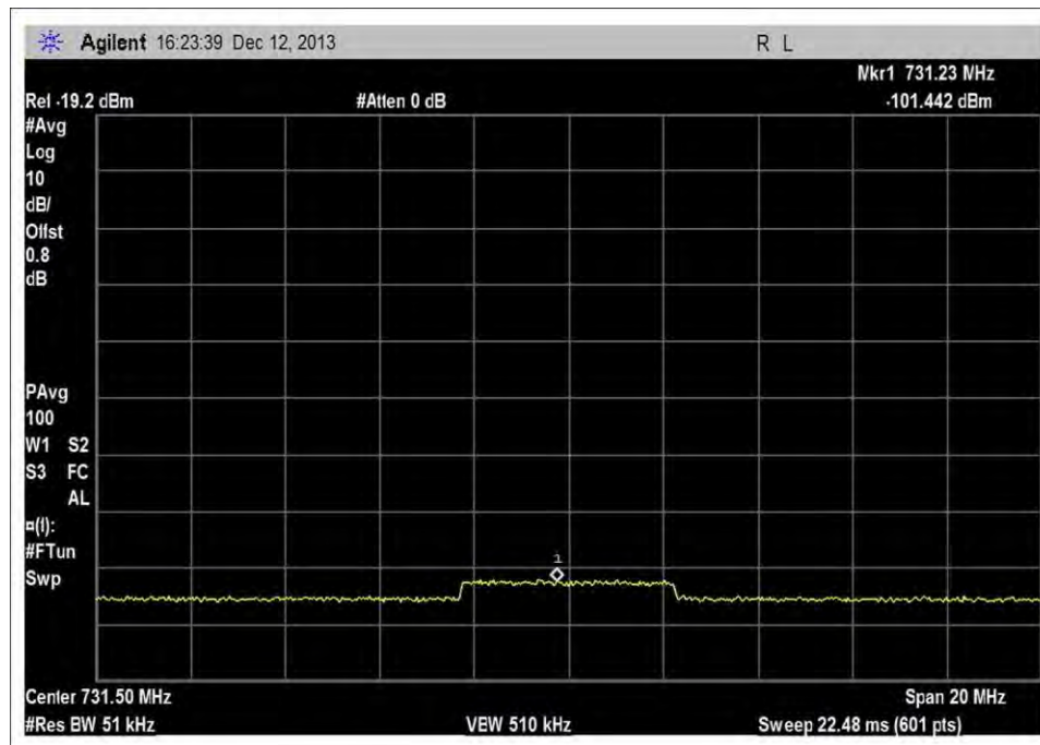
DL_716-746MHz_Input
