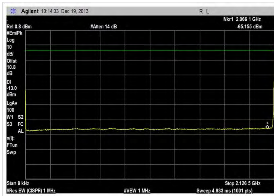
DL_2110-2155MHz_M_10LTE_1
