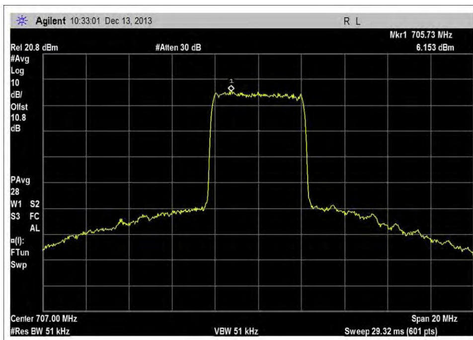
UL_698-716MHz_Output
