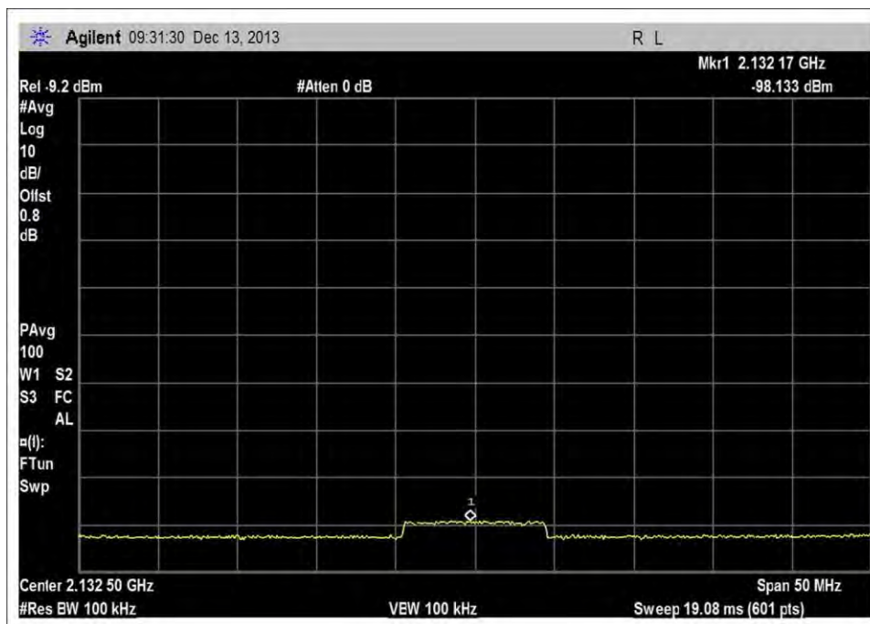
DL_2110-2155MHz_Input
