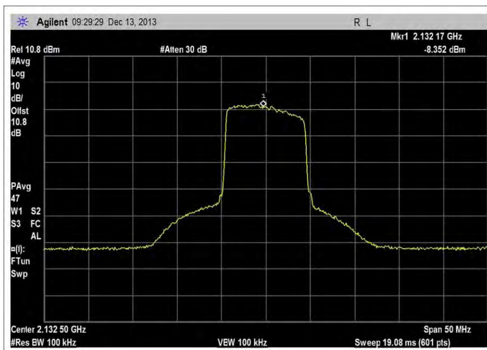
DL_2110-2155MHz_Output
