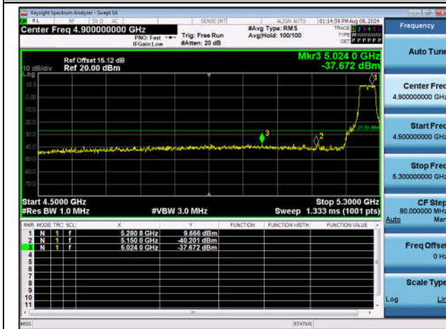
11N40SISO-Ant1-5270-PASS
